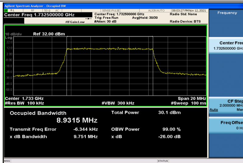
Band4-10MHz-QPSK-20175-50RB#0-8.9315
