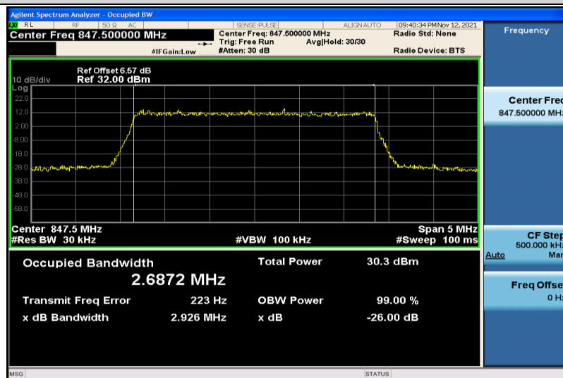
Band5-3MHz-QPSK-20635-15RB#0-2.6872
