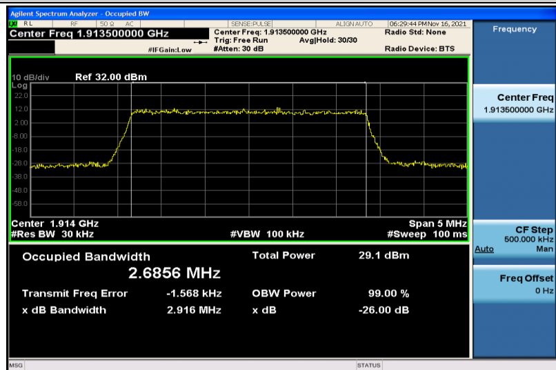
Band25-3MHz-QPSK-26675-15RB#0-2.6856
