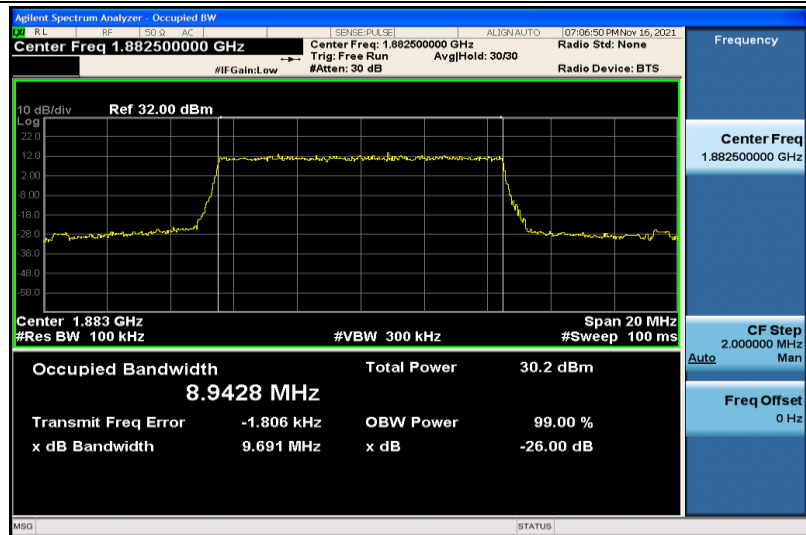
Band25-10MHz-QPSK-26365-50RB#0-8.9428
