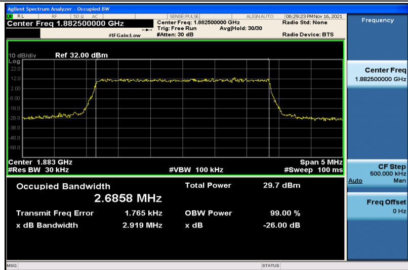
Band25-3MHz-QPSK-26365-15RB#0-2.6858
