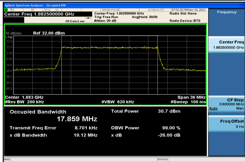
Band25-20MHz-QPSK-26365-100RB#0-17.859
