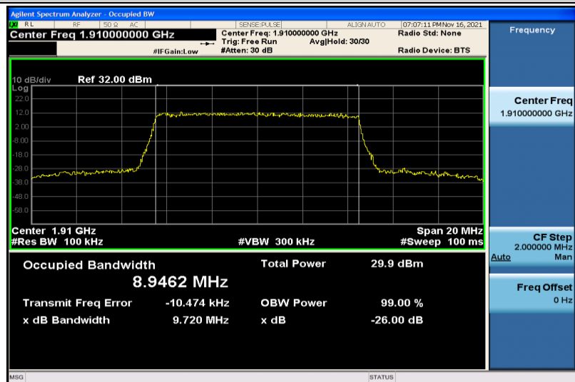
Band25-10MHz-QPSK-26640-50RB#0-8.9462
