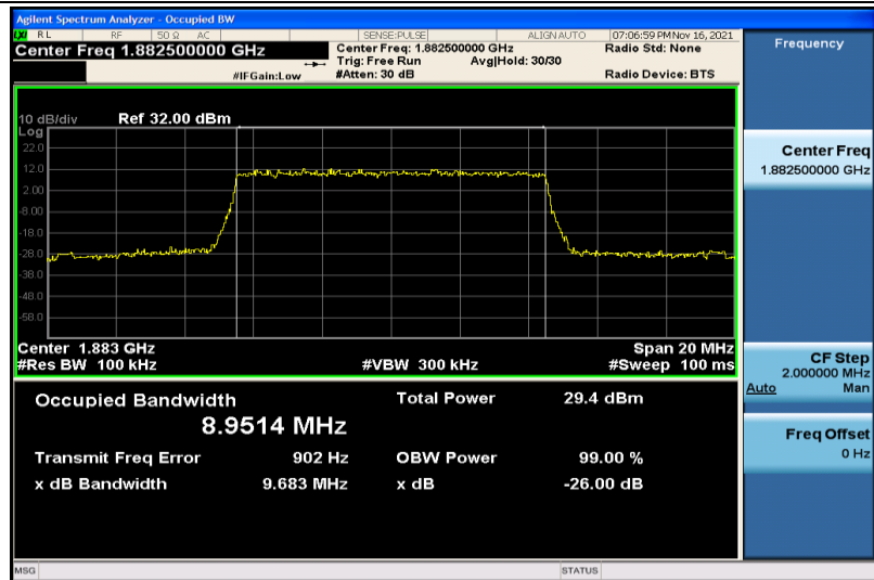
Band25-10MHz-16QAM-26365-50RB#0-8.9514
