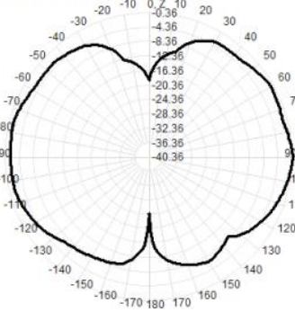
2500.0MHz Total(E2-YZ), Max=-0.39dBi
