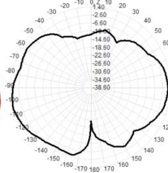
2400.0MHz Total(E1-XZ), Max= 1.40dBi
