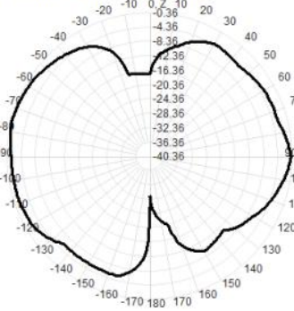
2500.0MHz Total(E1-XZ), Max=-0.56dBi
