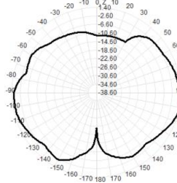
2400.0MHz Total(E2-YZ), Max= 0.93dBi
