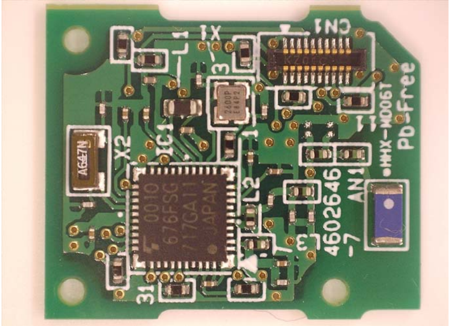
RF Module
