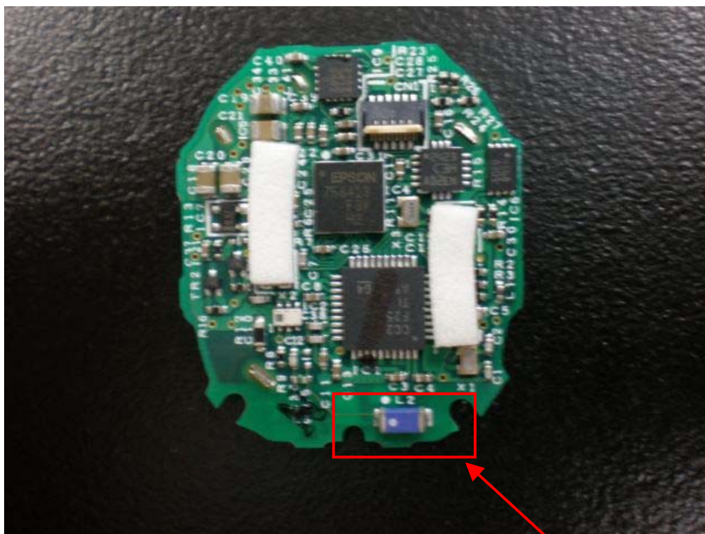
Antenna
