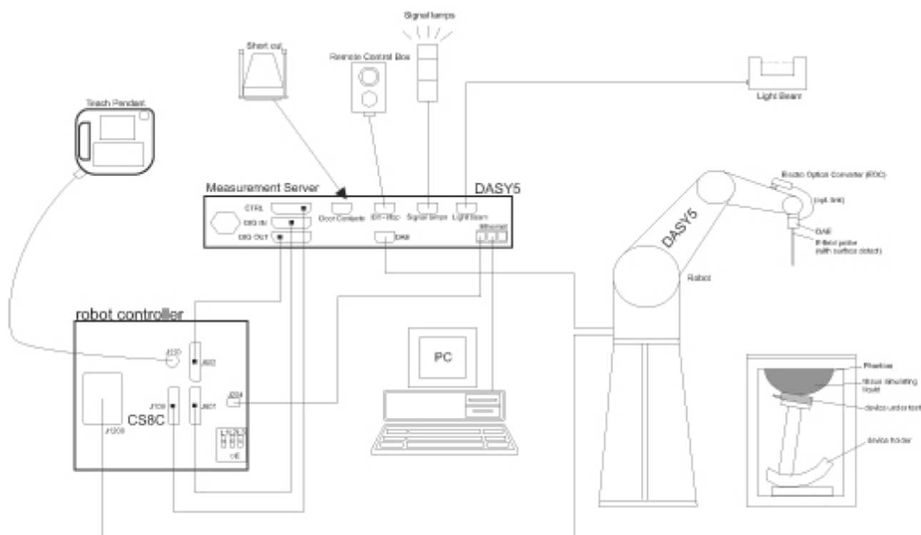
Fig. 5.1 DASY5 System
