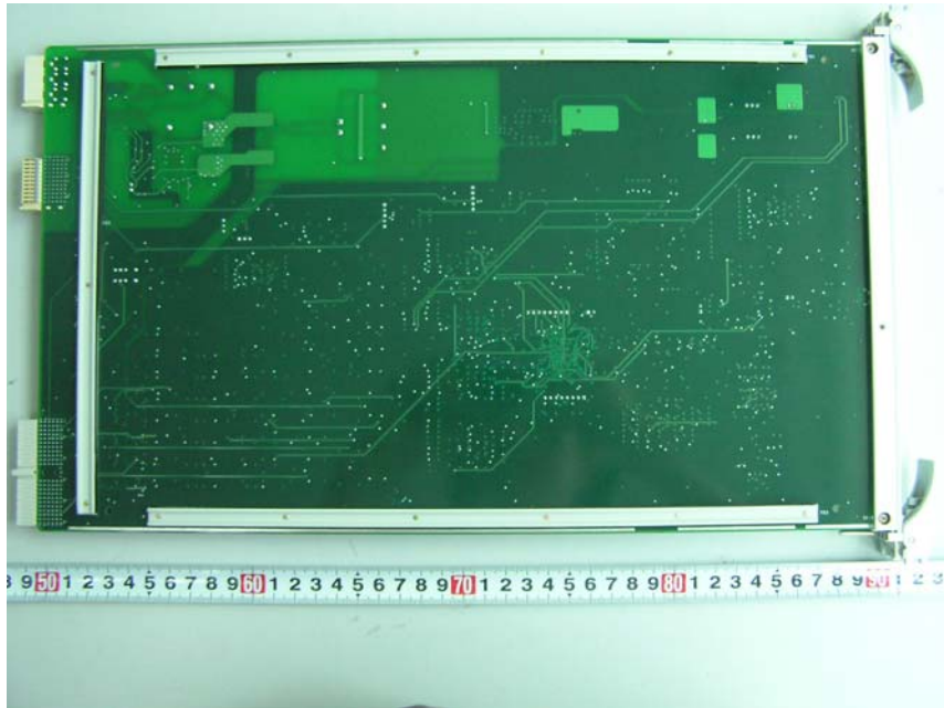
SAM PCB Bottom View
