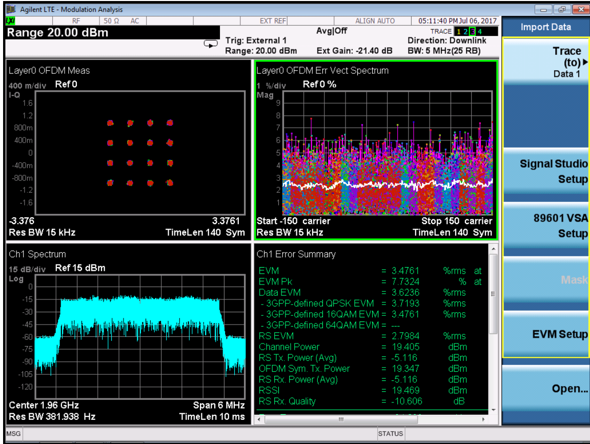
LTE 5M-Port 1-1960MHz-E-TM3.3
