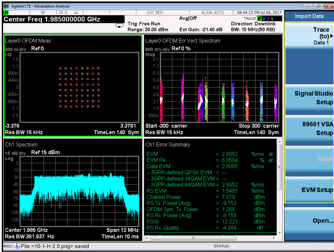
LTE 10M-Port 1-1985MHz-E-TM3.1
