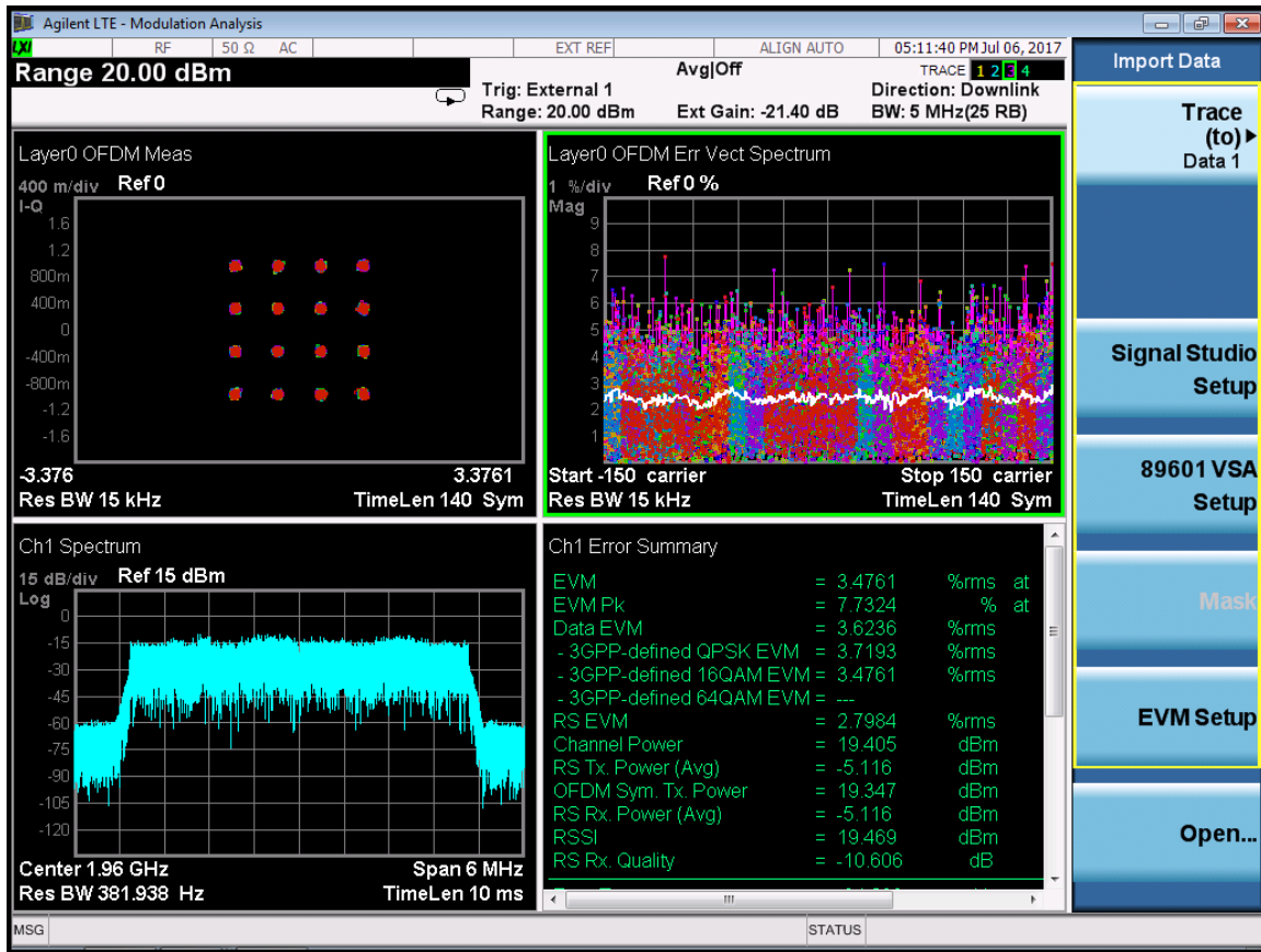
LTE 5M-Port 0-1960MHz-E-TM3.3
