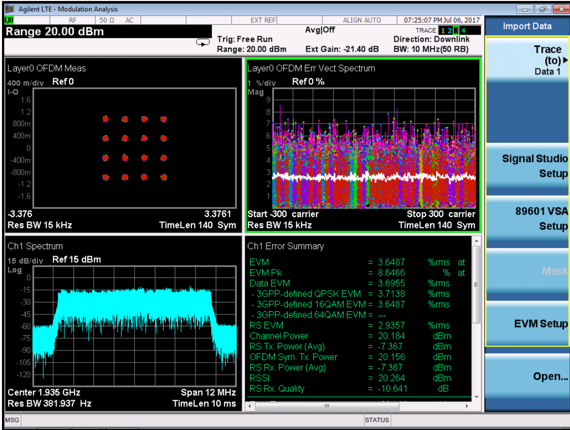
LTE 10M-Port 1-1935MHz-E-TM3.3
