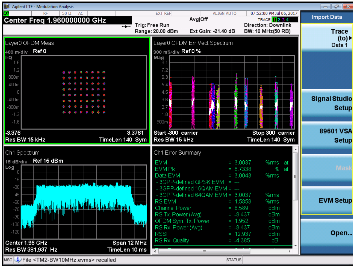
LTE 10M-Port 0-1960MHz-E-TM3.1
