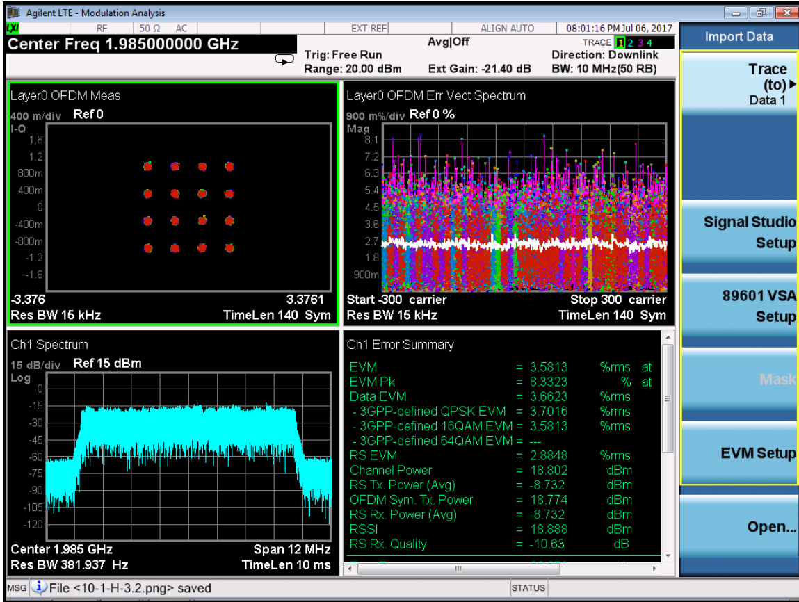
LTE 10M-Port 1-1985MHz-E-TM3.3
