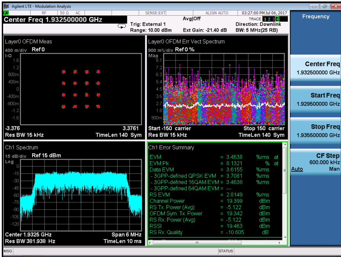
LTE 5M-Port 0-1932.5MHz-E-TM3.3
