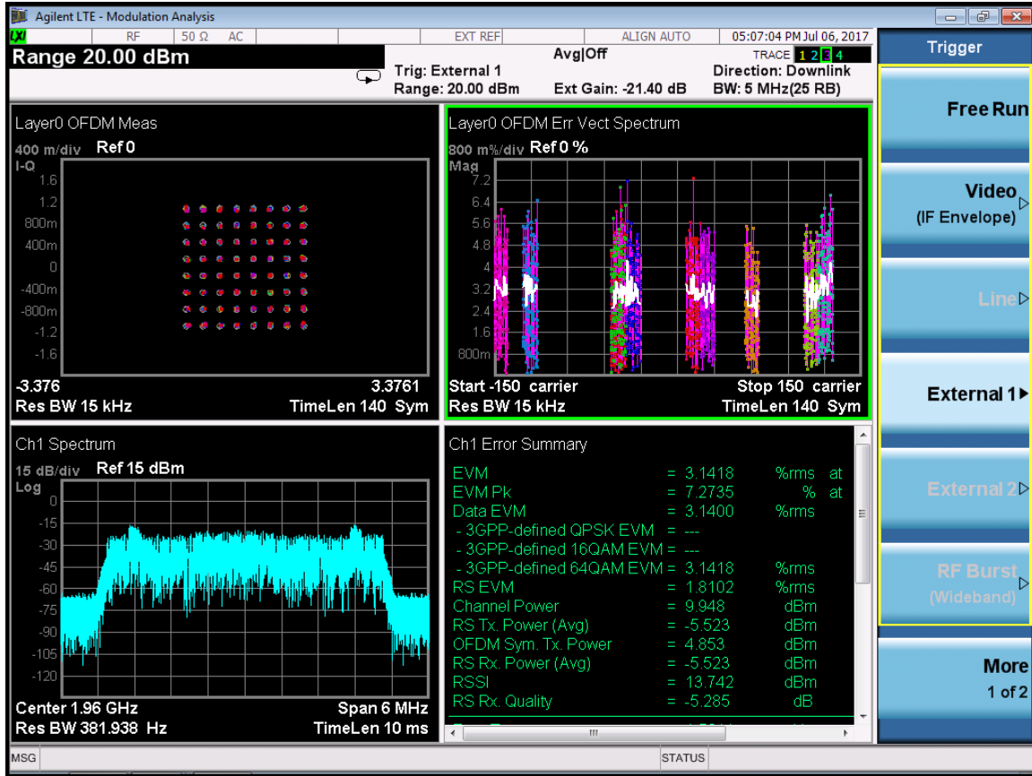
LTE 5M-Port 1-1960MHz-E-TM3.1
