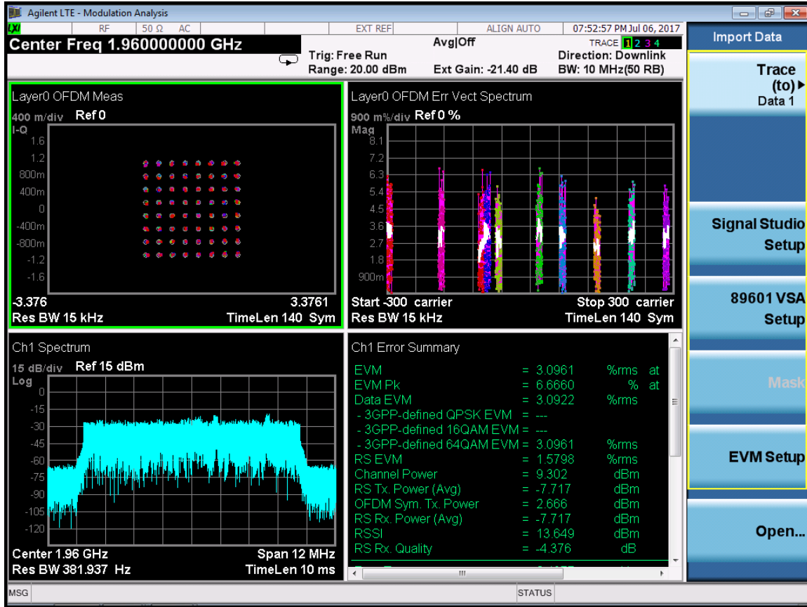
LTE 10M-Port 1-1960MHz-E-TM3.1
