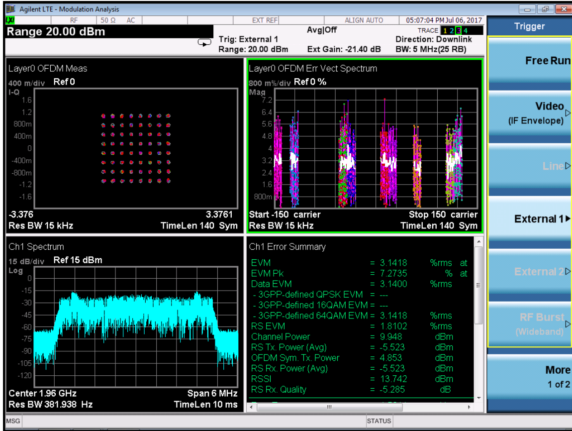
LTE 5M-Port 0-1960MHz-E-TM3.1
