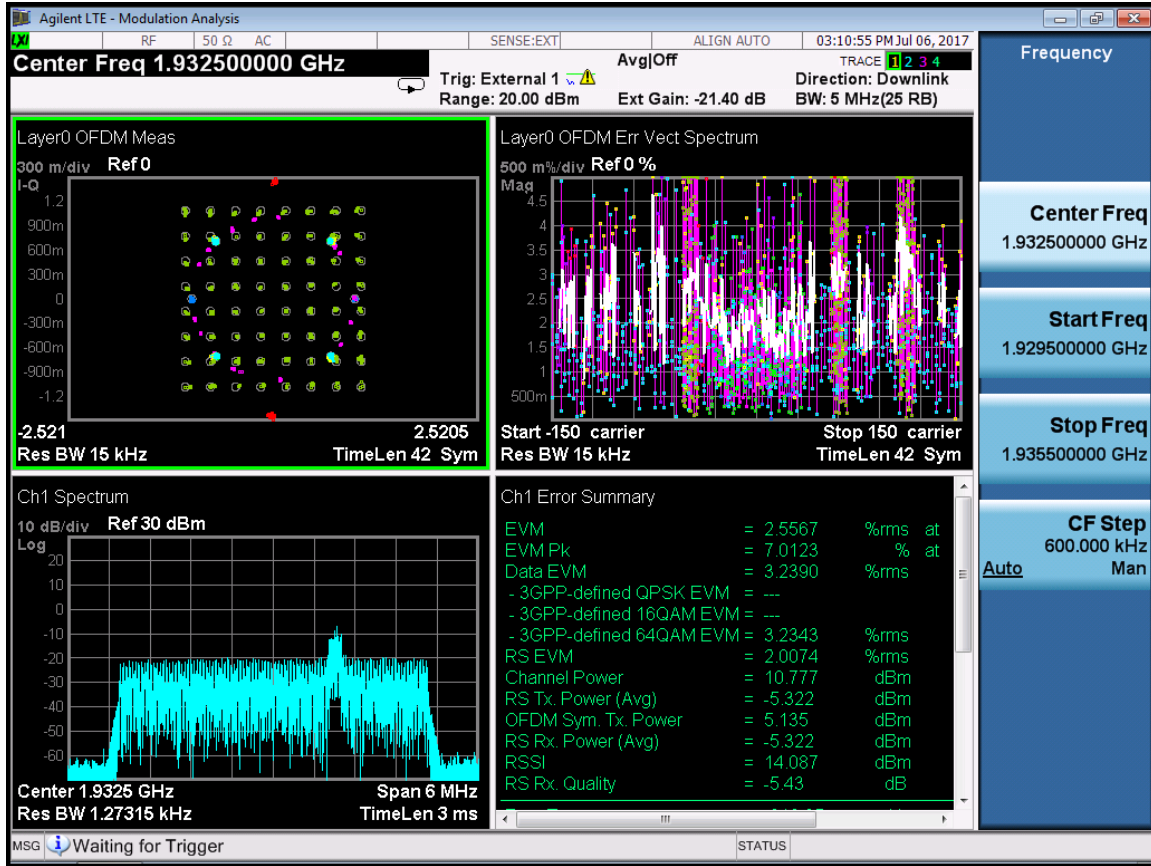
LTE 5M-Port 1-1932.5MHz-E-TM3.1
