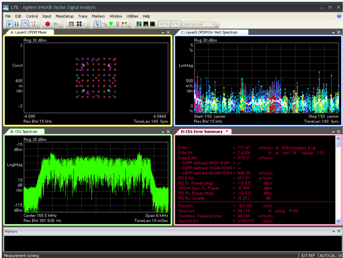
5M -Port 1 -765.5MHz-TM3.1
