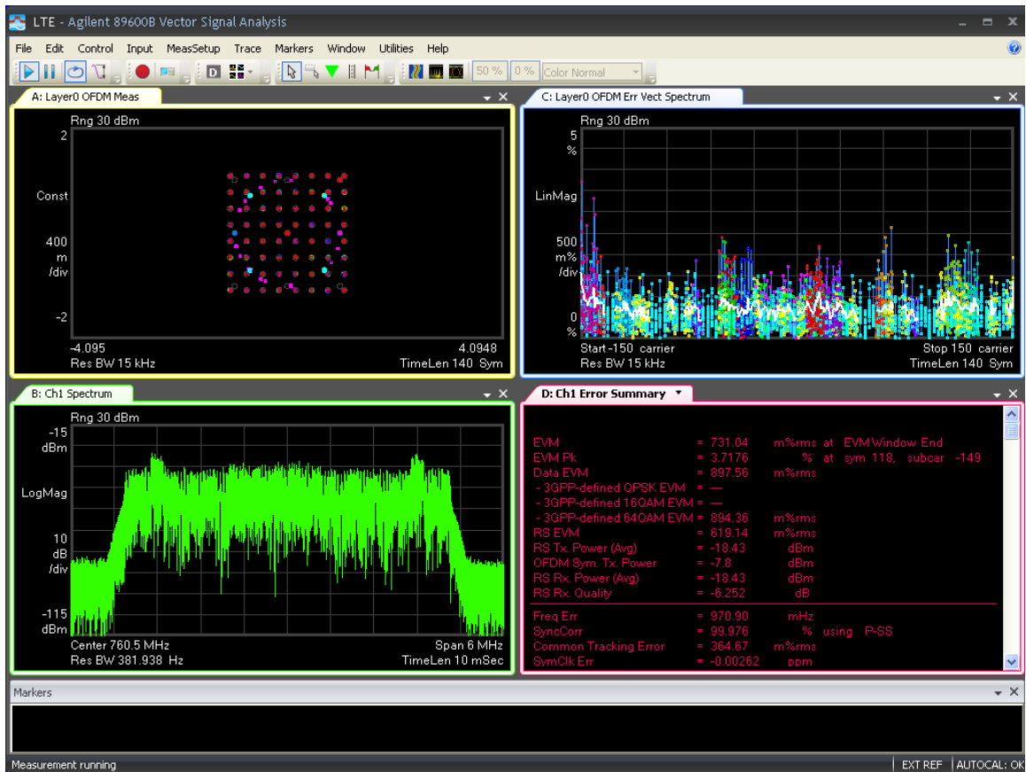
5M -Port 2 -760.5MHz-TM3.1
