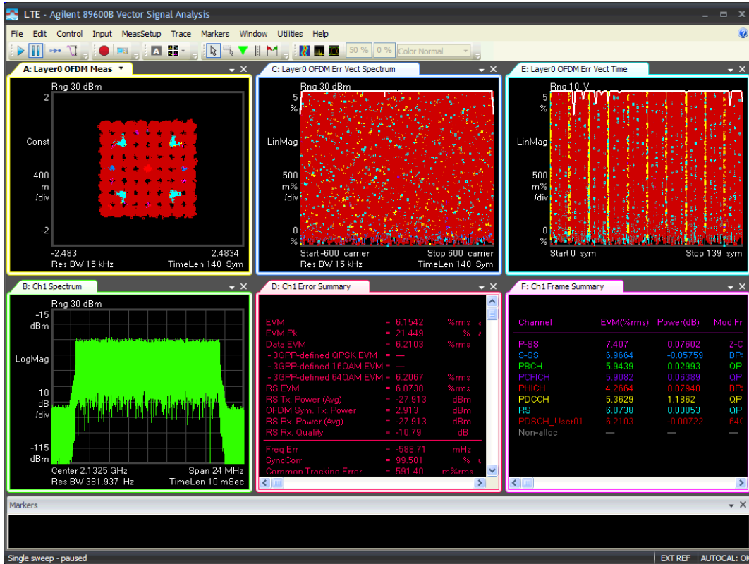
20M-Port 2 -2132.5MHz-TM3.2
