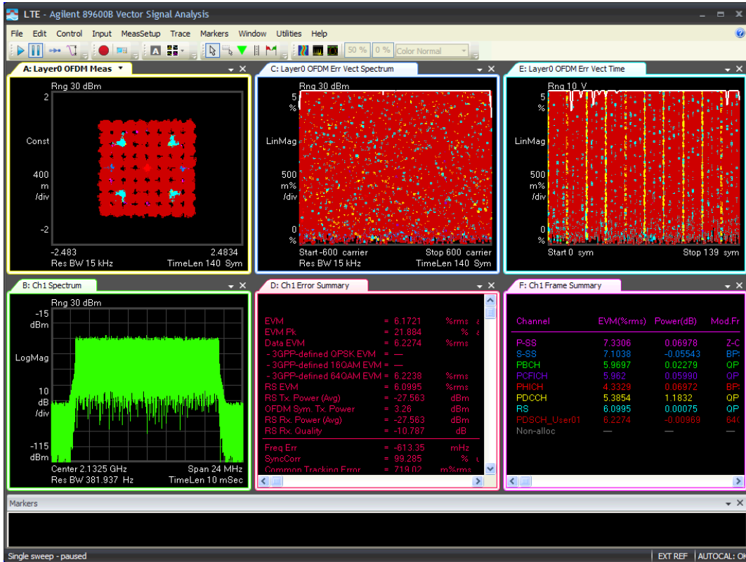
20M-Port 1 -2132.5MHz-TM3.2
