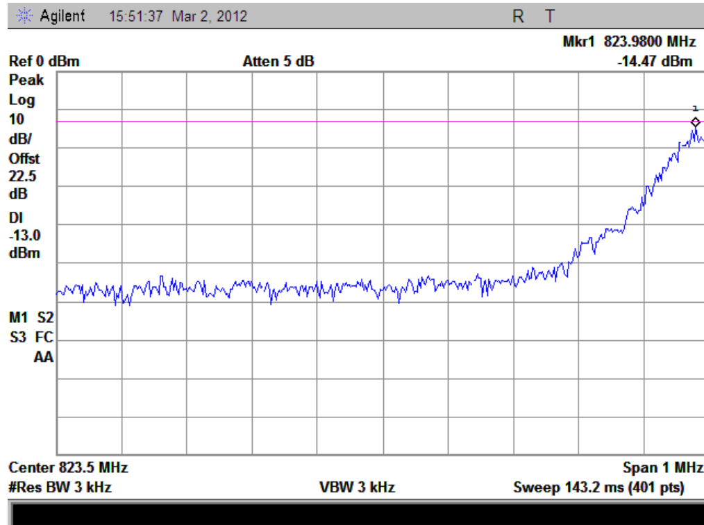
(Plot A: EDGE 850 Channel = 128)
