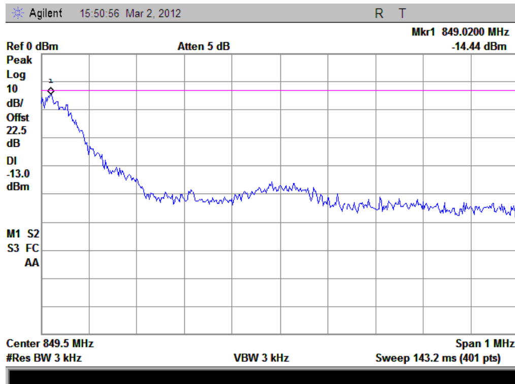
(Plot B: EDGE 850 Channel = 251)
