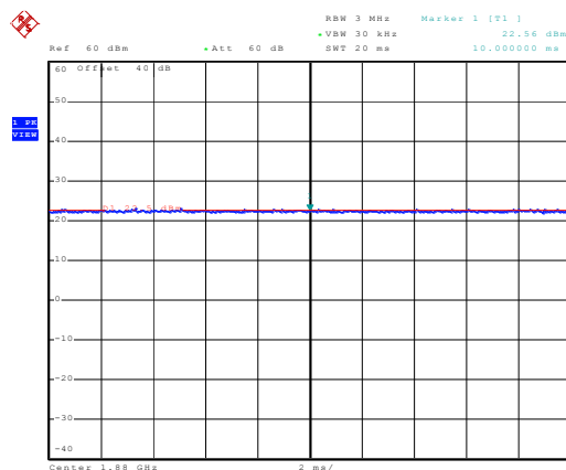
1880MHz - WCDMA
