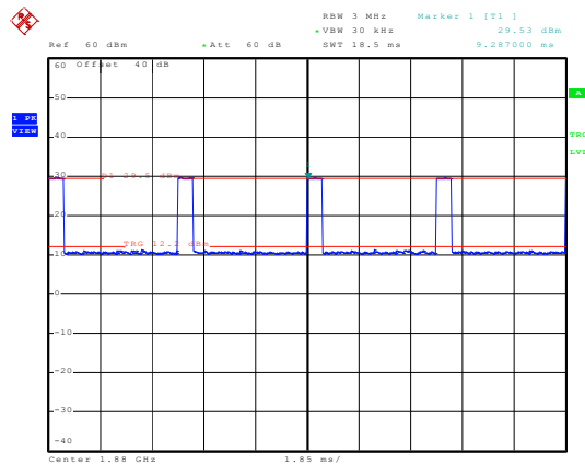
1880MHz - GSM
