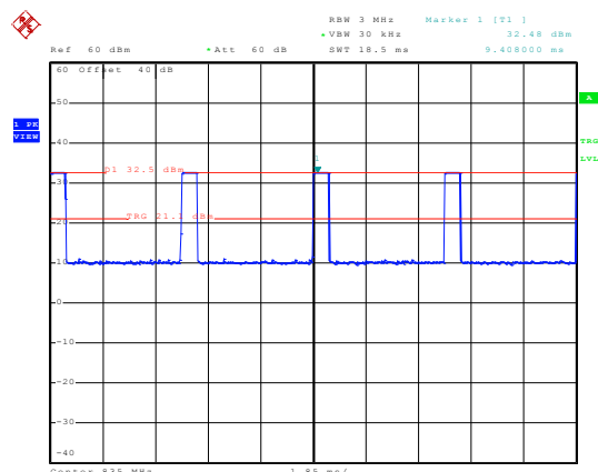
835MHz - GSM
