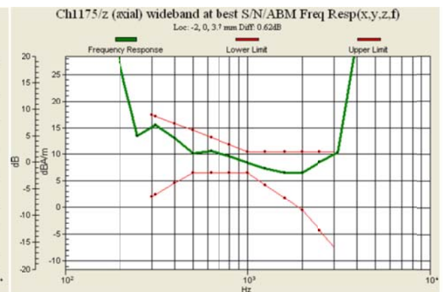
Fig. 8.6 CDMA2000 BC1 Ch1175
