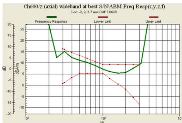
Fig. 8.5 CDMA2000 BC1 Ch600
