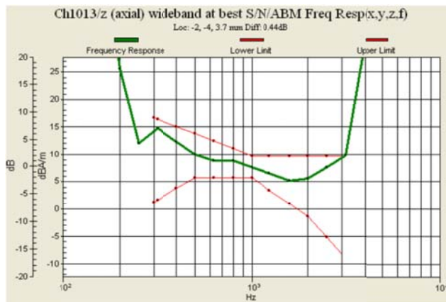
Fig. 8.1 CDMA2000 BC0 Ch1013
