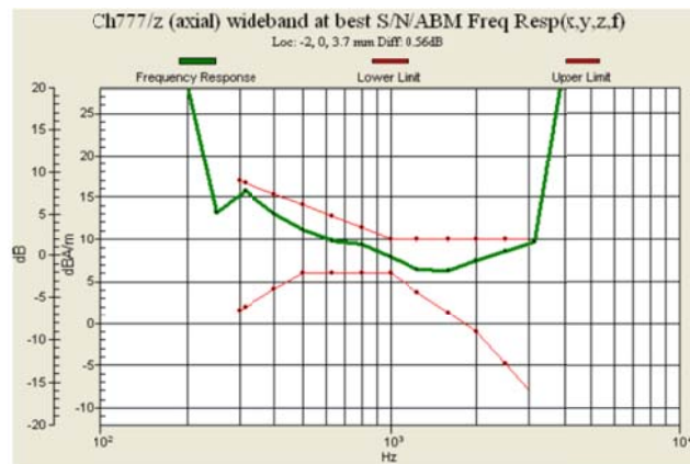
Fig. 8.3 CDMA2000 BC0 Ch777
