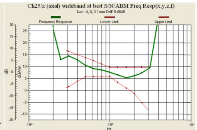
Fig. 8.4 CDMA2000 BC1 Ch25
