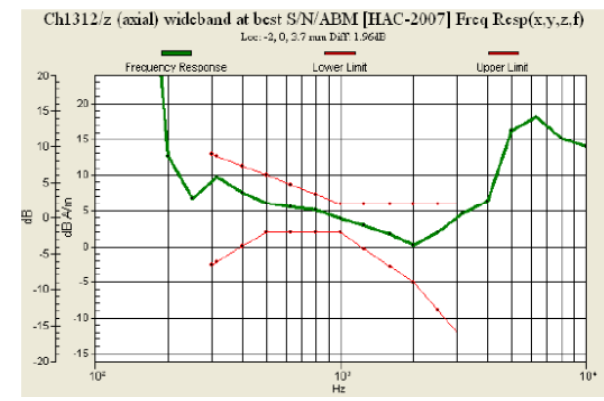
Fig. 9.4 WCDMA Band IV Ch1312
