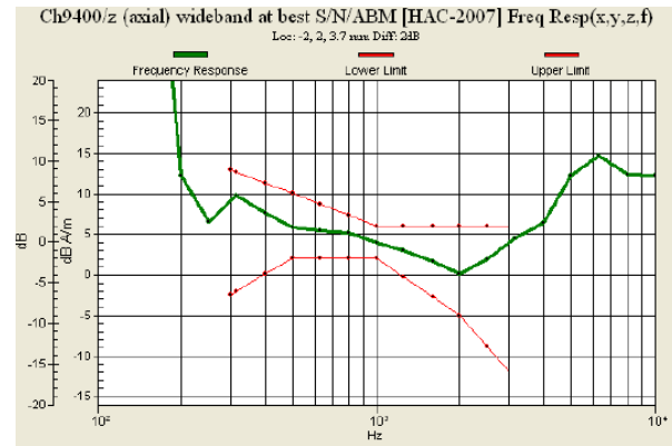
Fig. 9.2 WCDMA Band II Ch9400
