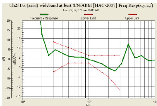
Fig. 9.3 GSM850 Ch251
