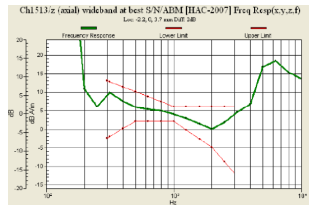
Fig. 9.6 WCDMA Band IV Ch1513
