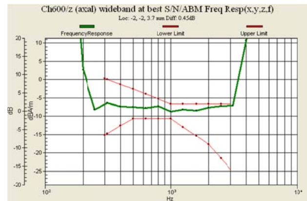
Fig 8.2 CDMA2000 BC1 Ch600
