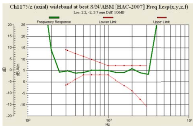
Fig. 9.3 CDMA2000 BC1 Ch1175
