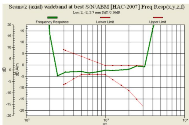
Fig. 9.7 CDMA2000 BC1 Ch25
