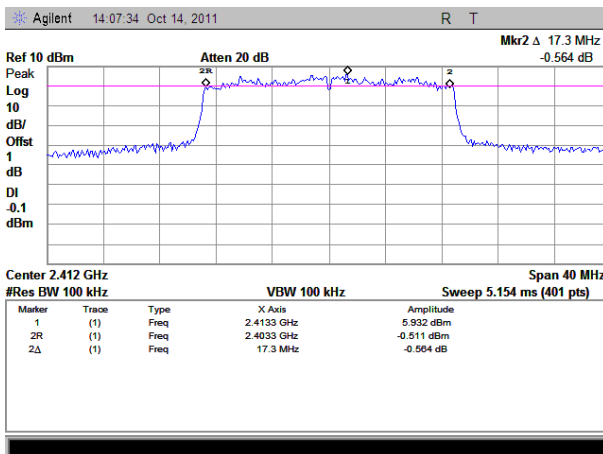
(Plot A: Chain1_Channel 1: 2412MHz)
