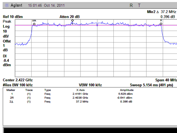
(Plot A: Chain1_Channel 3: 2422MHz)
