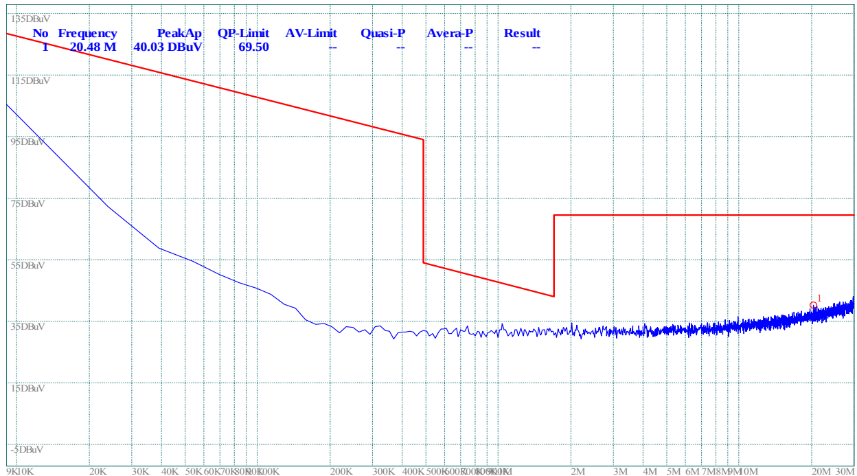
(Plot A: 9K – 30M)
