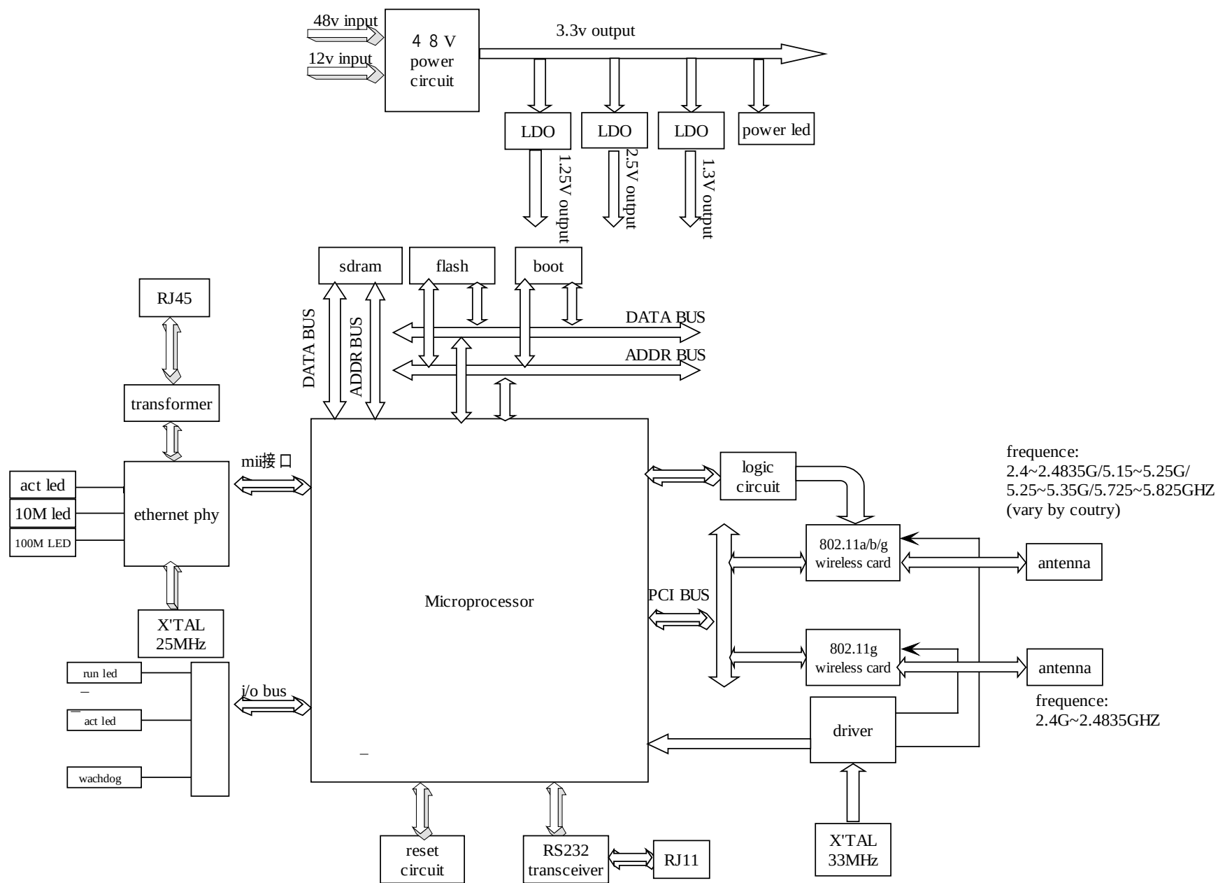
W800A 原理图
