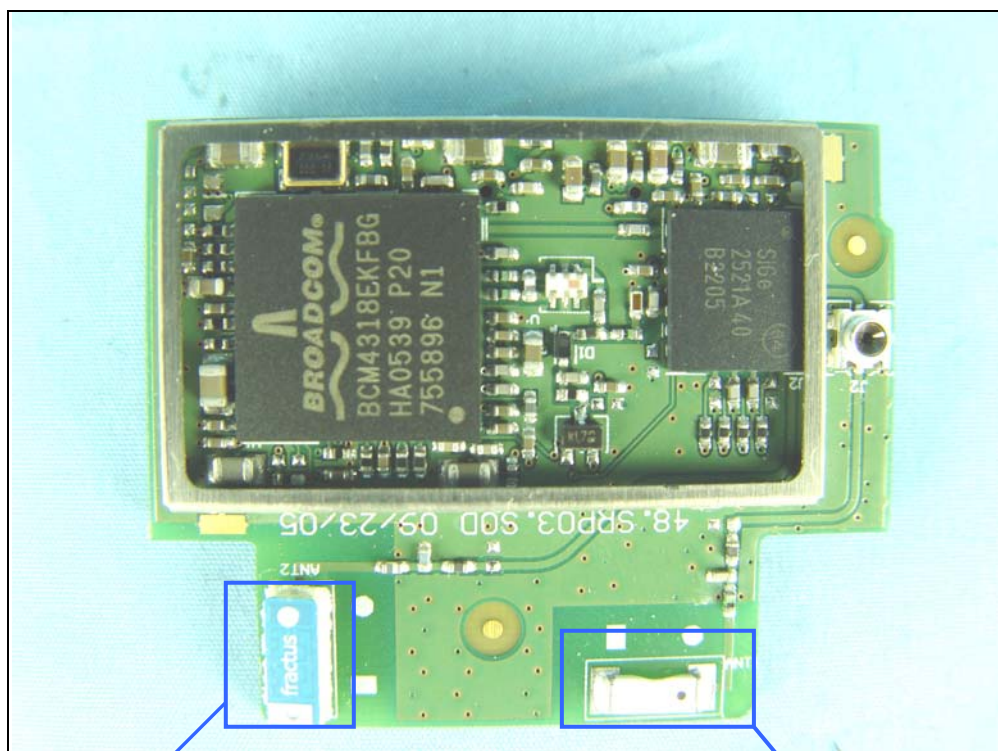
Aux. antenna
