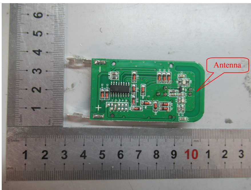
EUT(BH18C) – PCB Bottom View
