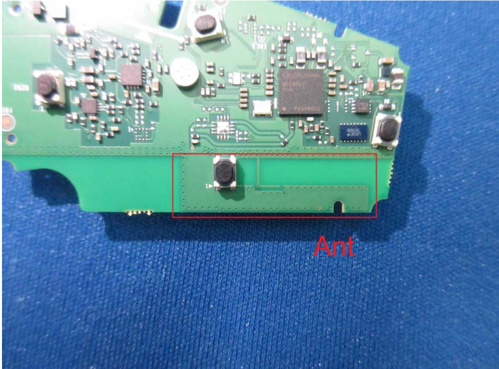
(8) EUT Photo (Antenna)
