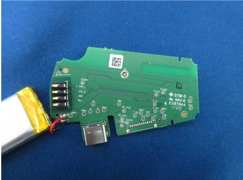
(10) EUT Photo
