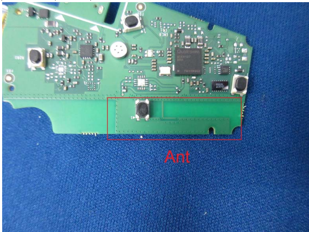
(21) EUT Photo (Antenna)
