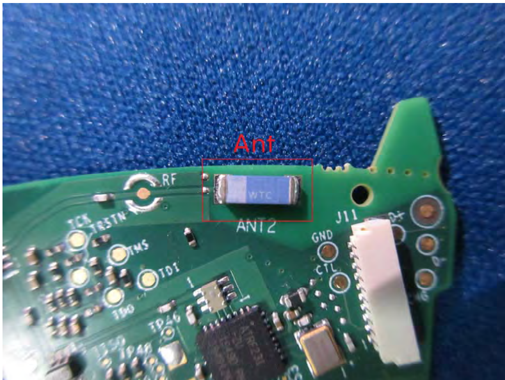
(8) EUT Photo (PIFA ANT)
