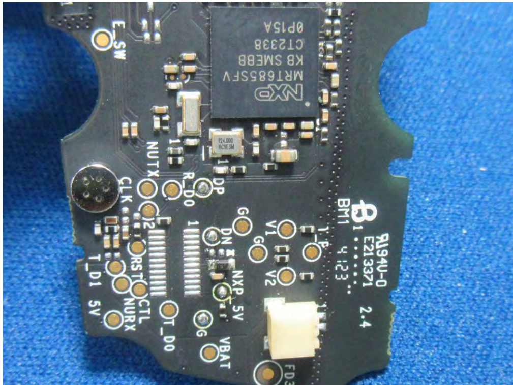
(8) EUT Photo (BT BR + EDR & BLE Antenna)
