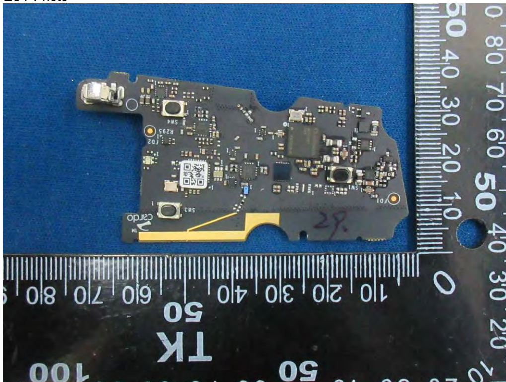
(4) EUT Photo
