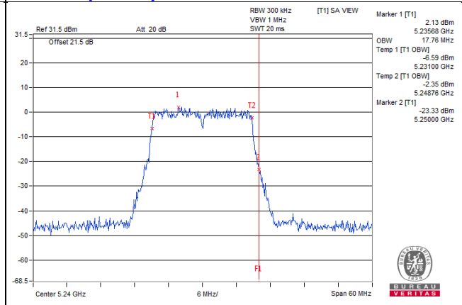
802.11ac(VHT20)_Chain1 / CH48
