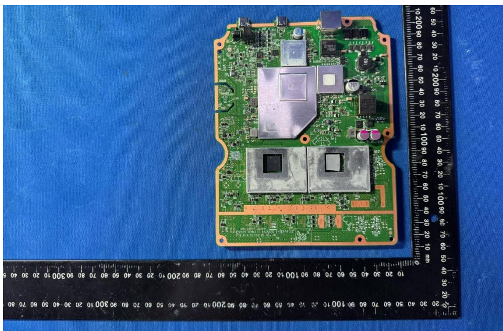
(30) EUT Photo
