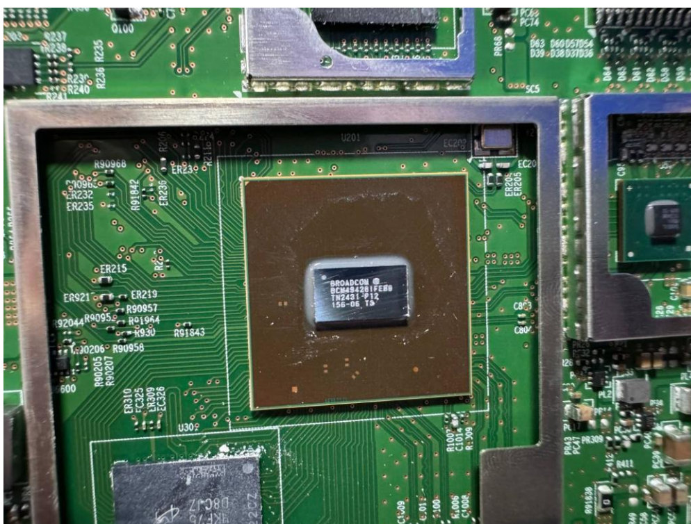
(36) EUT Photo
