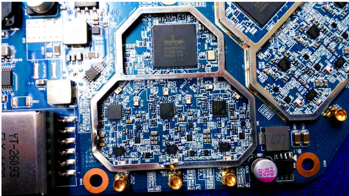
5G WIFI Module
