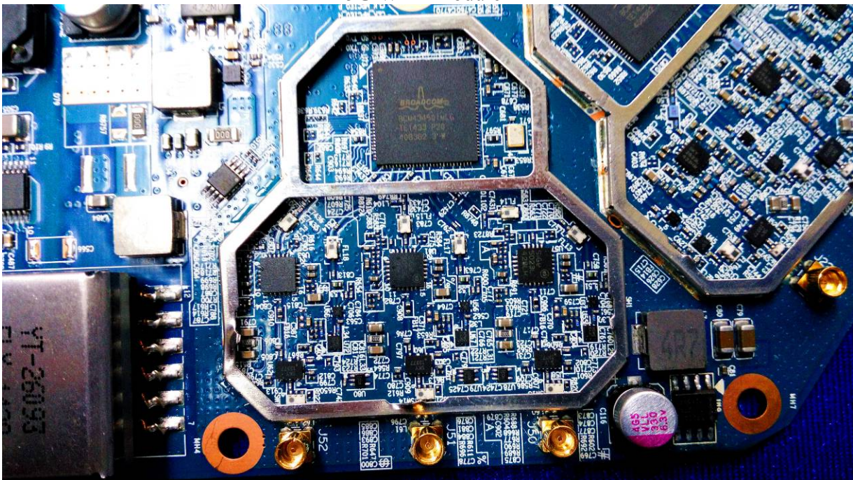
5G WIFI Module
