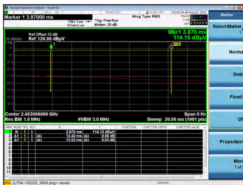
802.11b Antenna 1+2
