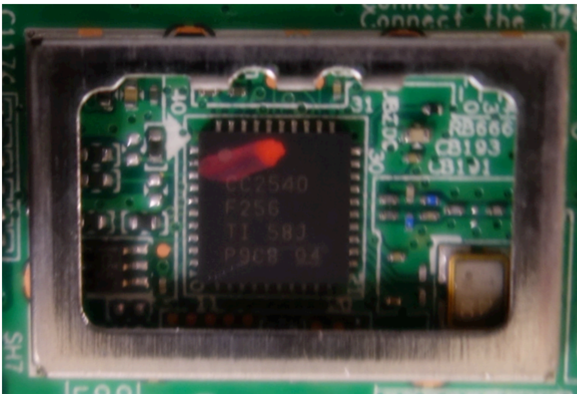
Close-Up BLE Chipset
