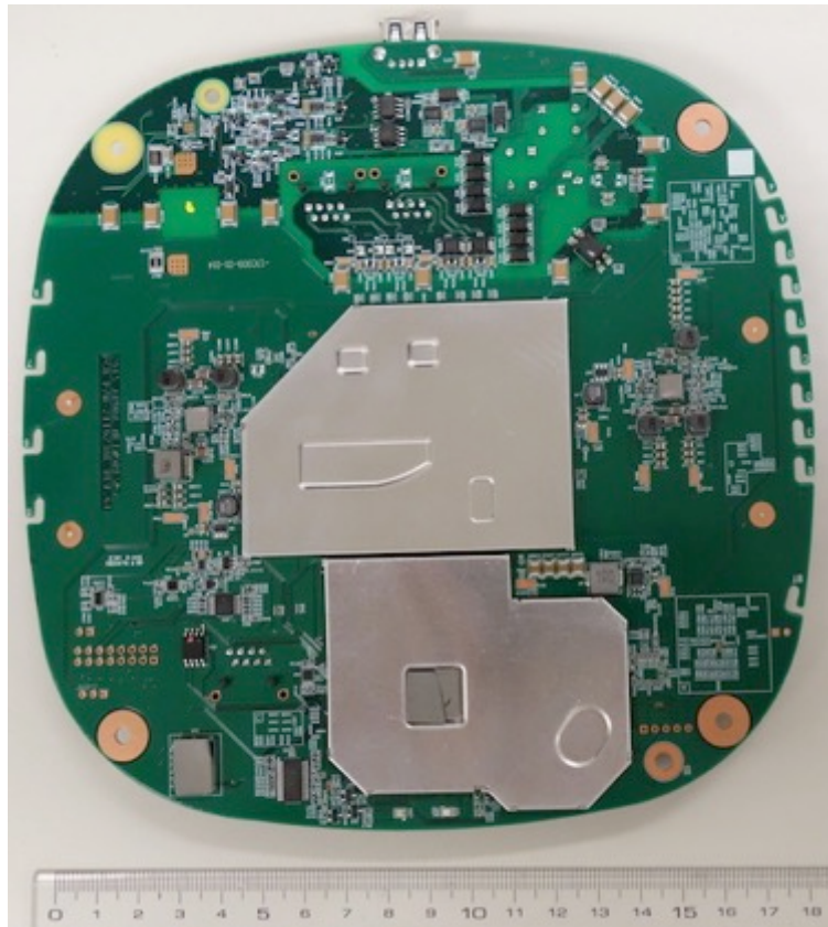
PCB - Bottom
