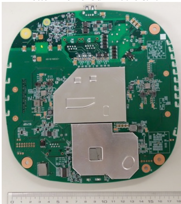
PCB - Bottom
