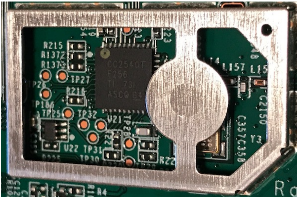
Close-Up: BLE
