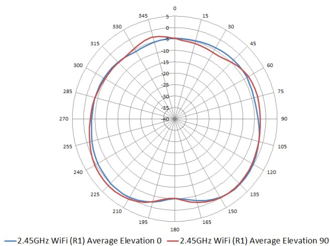
2.45GHz Wi-Fi (antennas 1, 2)
