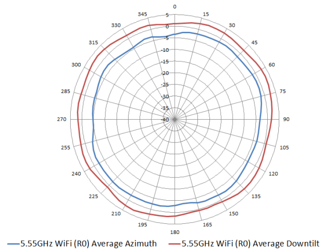
5.55GHz Wi-Fi (antennas 1, 2)
