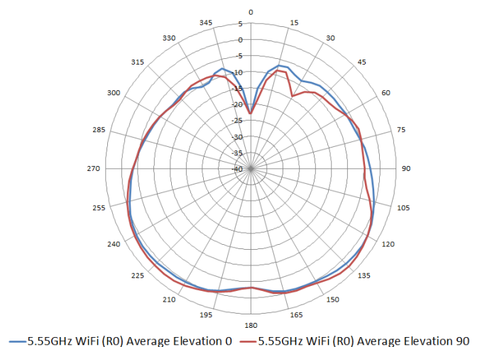
5.55GHz Wi-Fi (antennas 1, 2)
