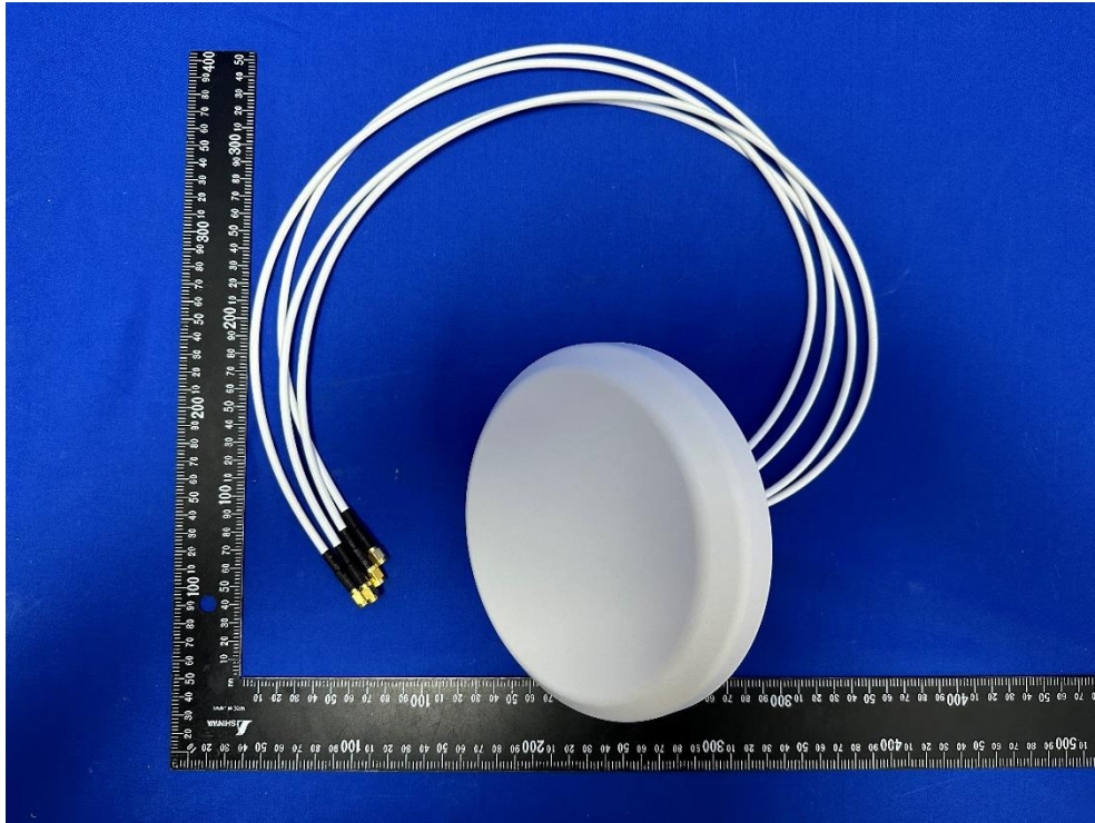
(11) EUT Photo - AP-ANT-340
