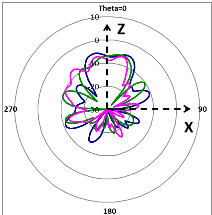
XZ_Pol._Theta_Ant.6
