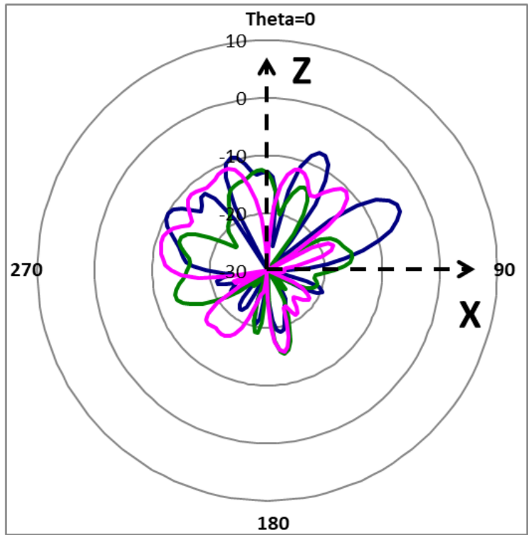
XZ_Pol._Theta_Ant.5
