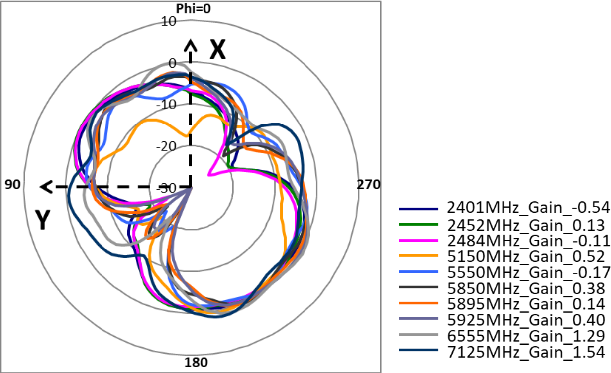
XY_Pol._Theta_Ant.9
