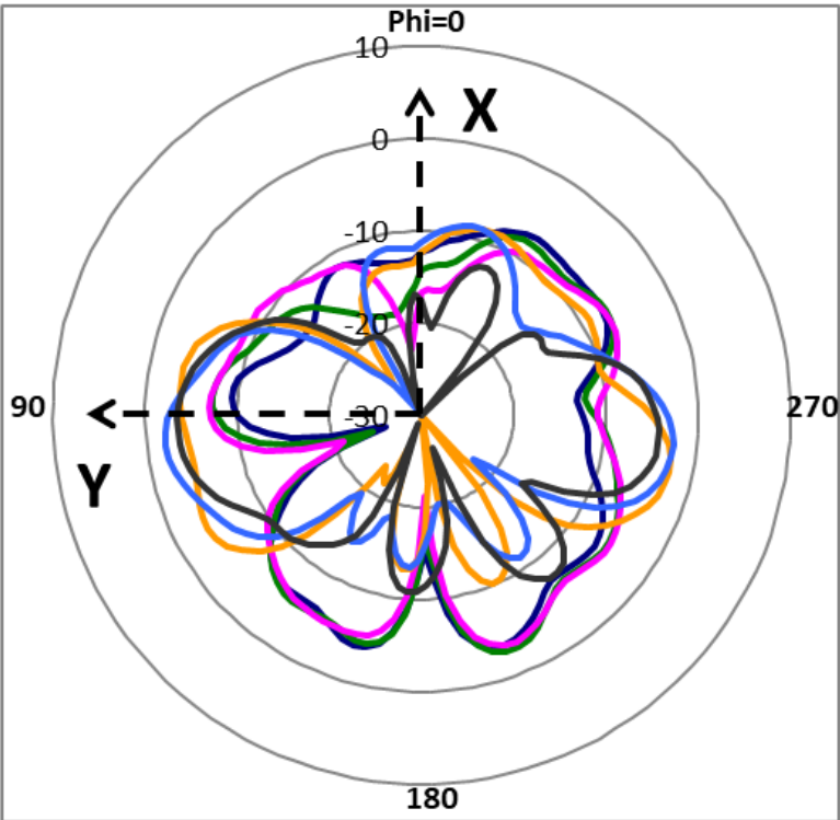
XY_Pol._Phi_Ant.8
