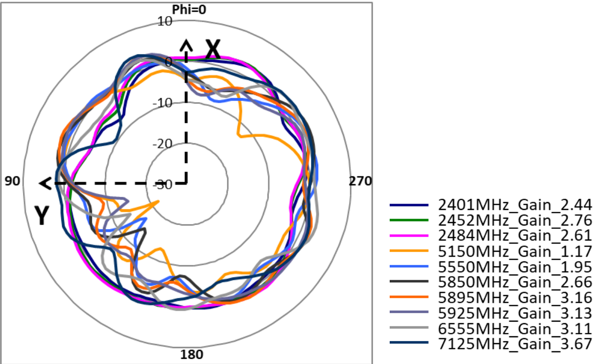
XY_Pol._Theta_Ant.12
