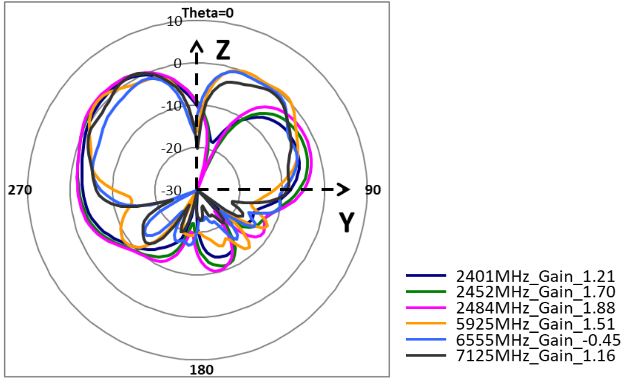
YZ_Pol._Theta_Ant.7
