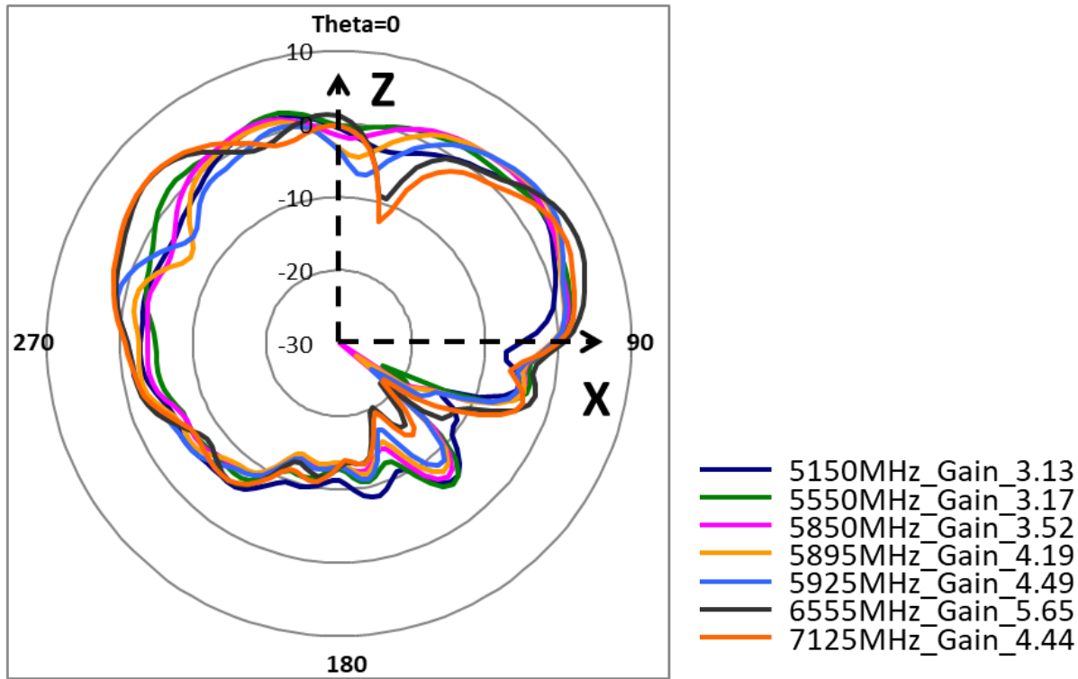
XZ_Pol._Theta_Ant.2
