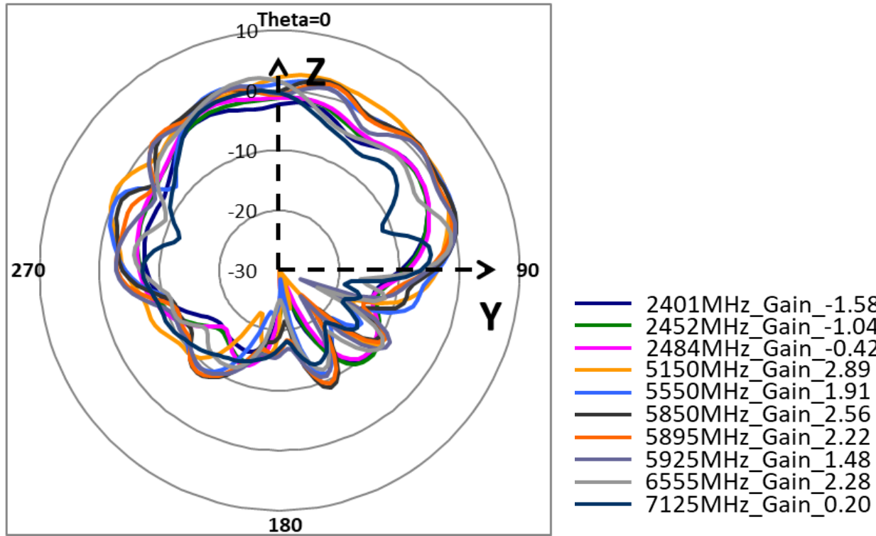
YZ_Pol._Phi_Ant.12
