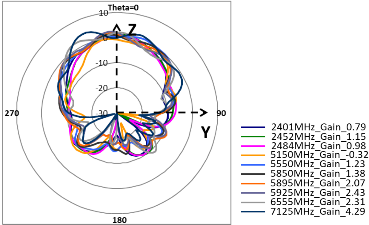
YZ_Pol._Theta_Ant.9
