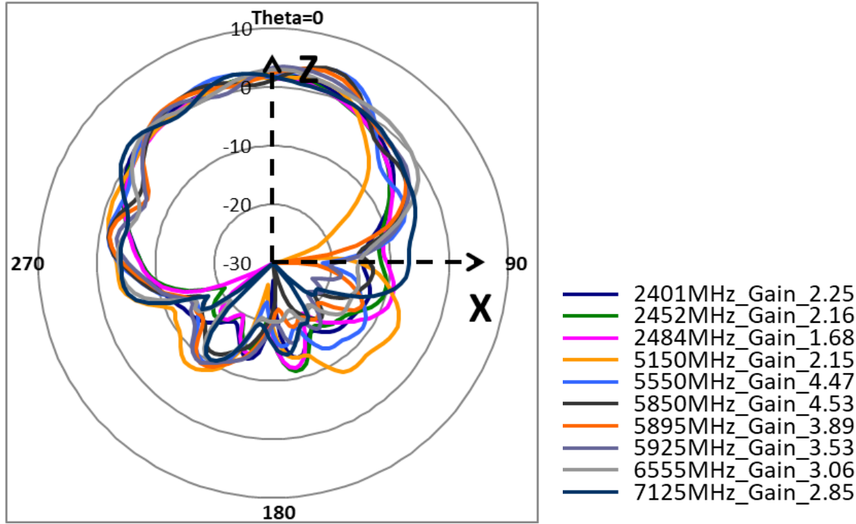
XZ_Pol._Theta_Ant.9
