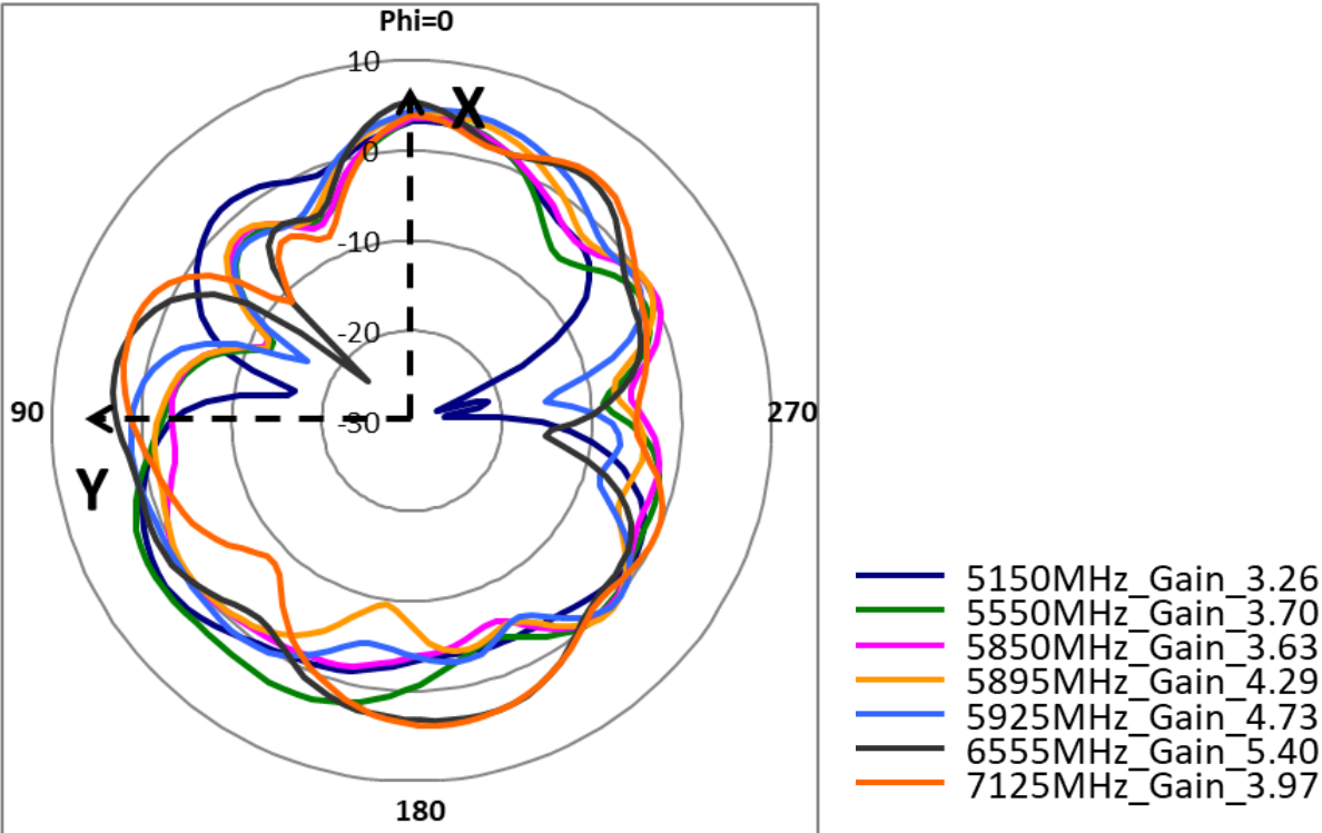
XY_Pol._Theta_Ant.2
