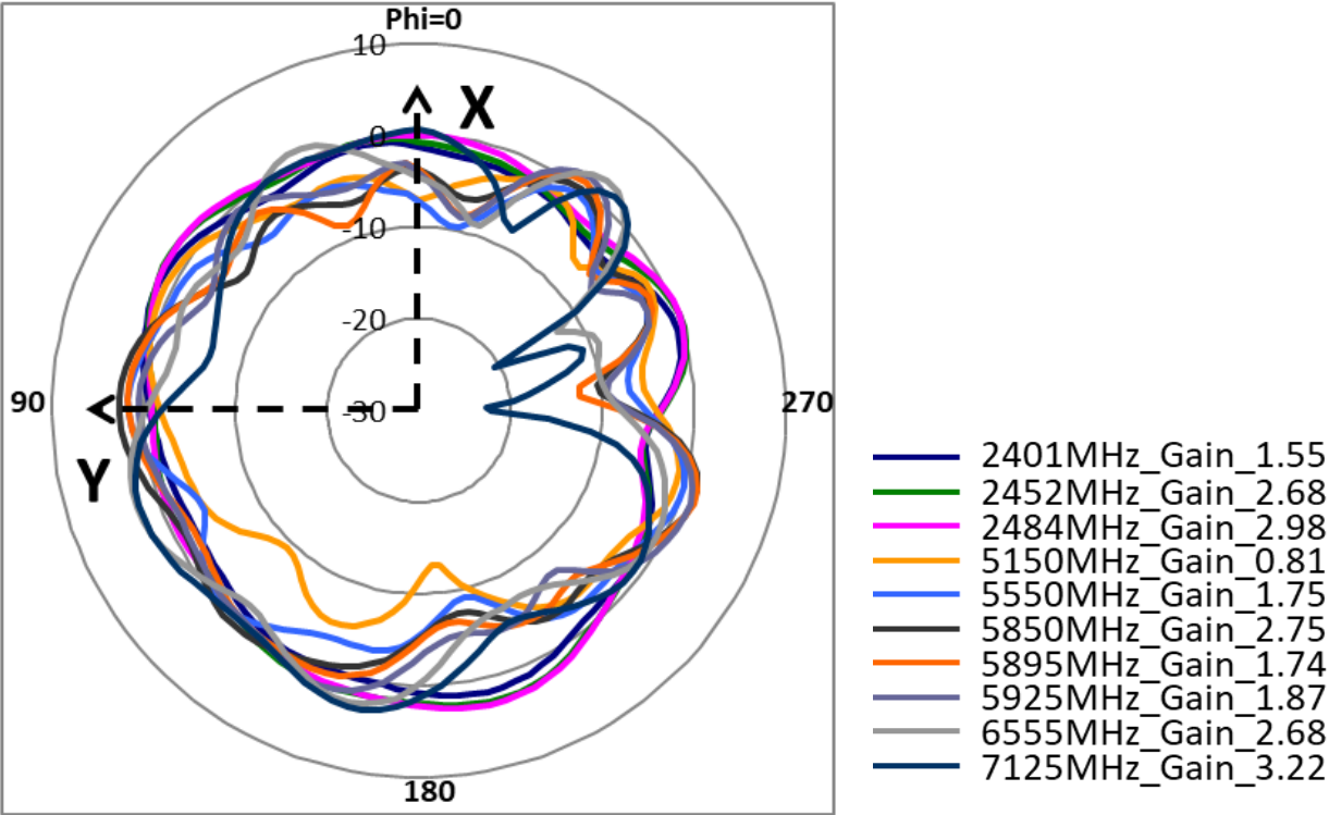
XY_Pol._Theta_Ant.11
