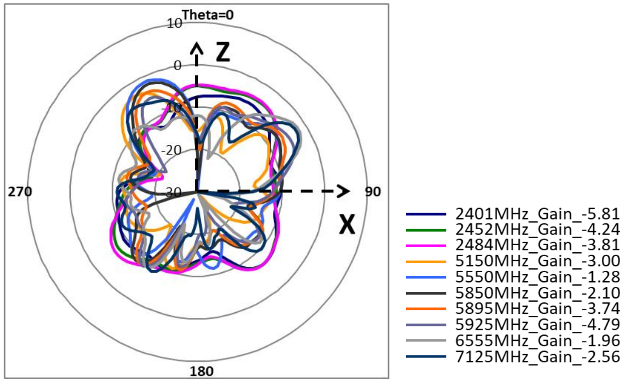
XZ_Pol._Phi_Ant.12
