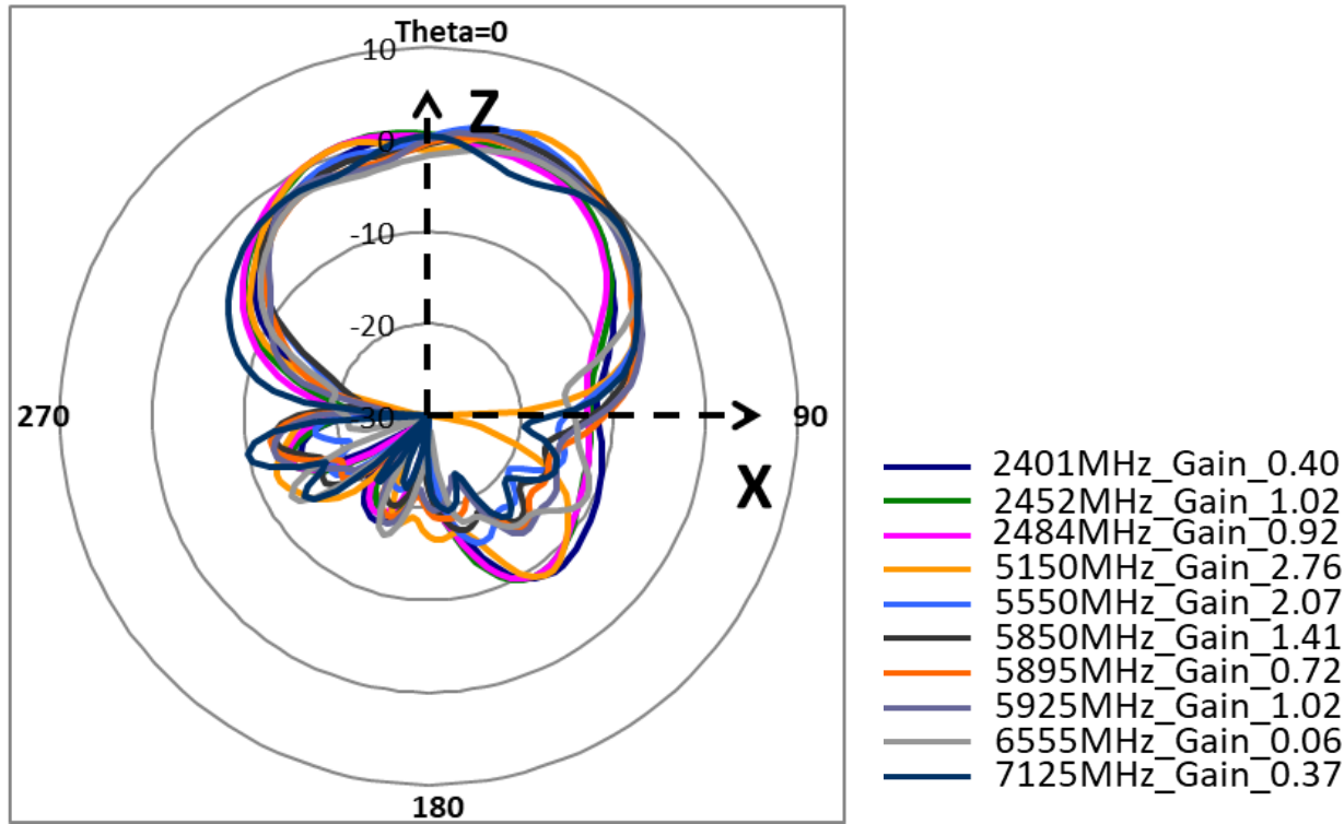
XZ_Pol._Theta_Ant.10
