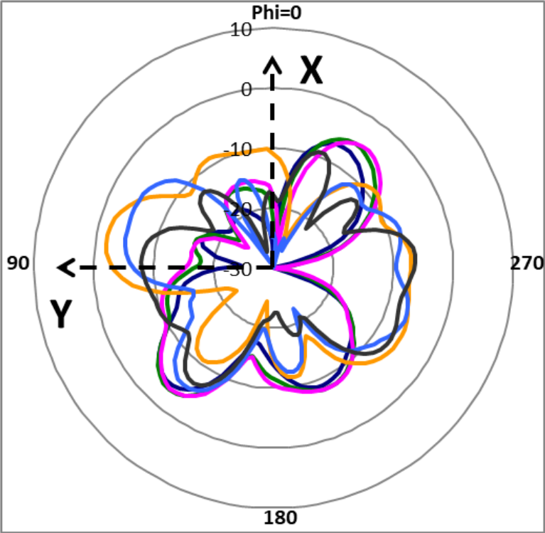
XY_Pol._Phi_Ant.7
