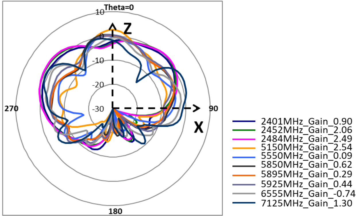
XZ_Pol._Theta_Ant.11
