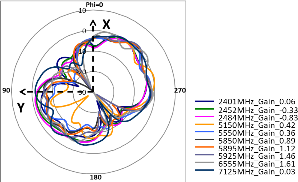
XY_Pol._Theta_Ant.10
