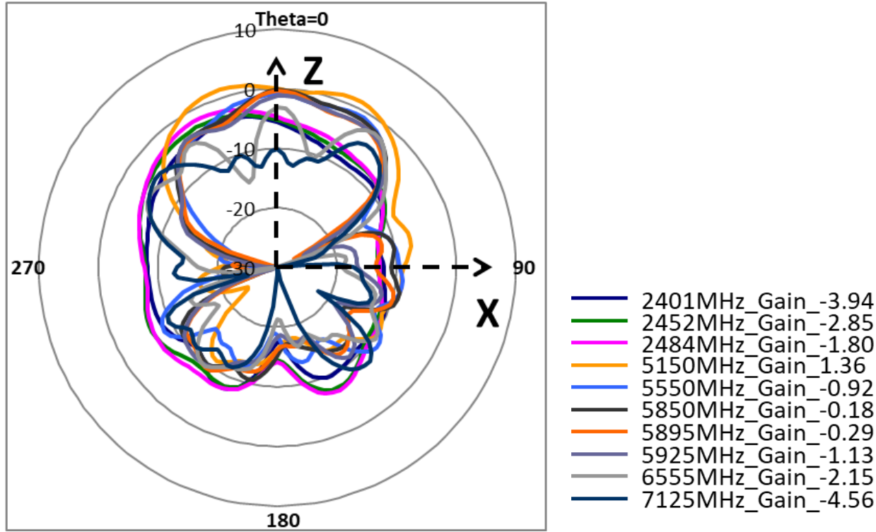
XZ_Pol._Phi_Ant.11
