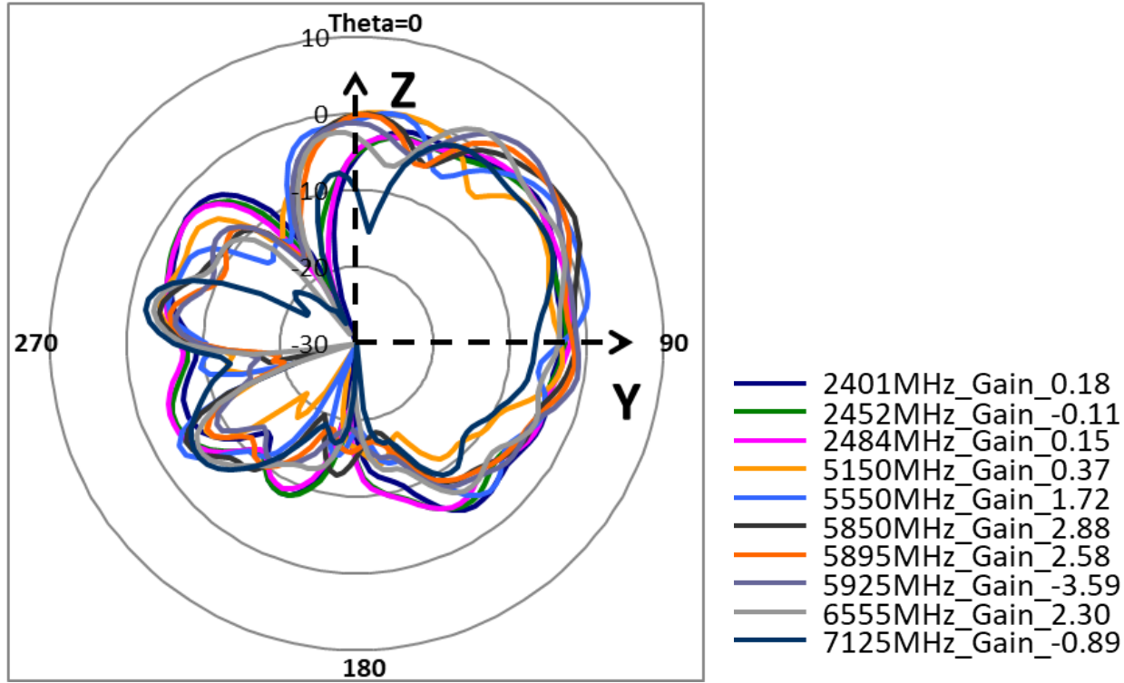
YZ_Pol._Theta_Ant.11
