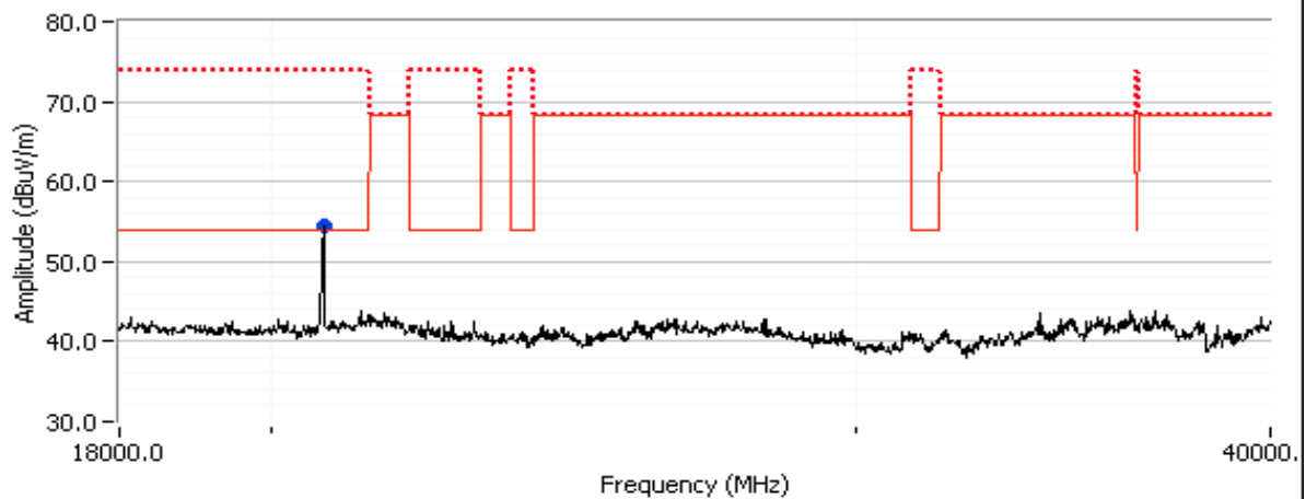
5180 MHz, 802.11n20 & 2412 MHz, 802.11b
