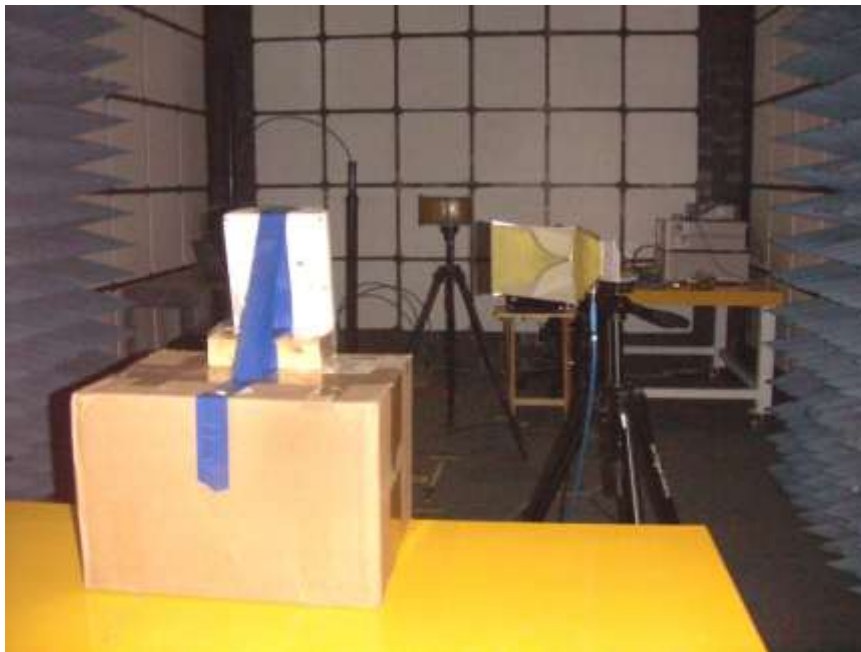
EUT BACK PHOTO
