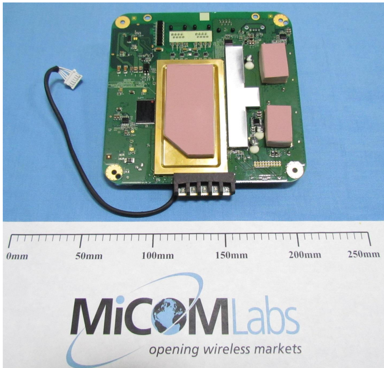
Bottomside - Radio-Board P/N: 13029025-701
