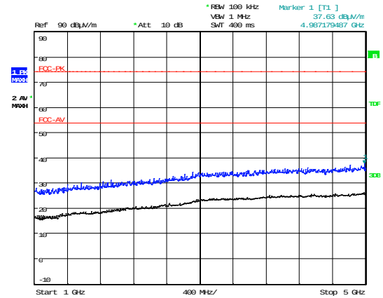
1GHz – 5GHz
