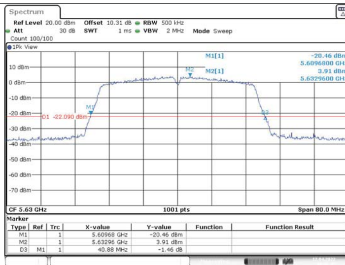
11N40MIMO_Ant2_5630
