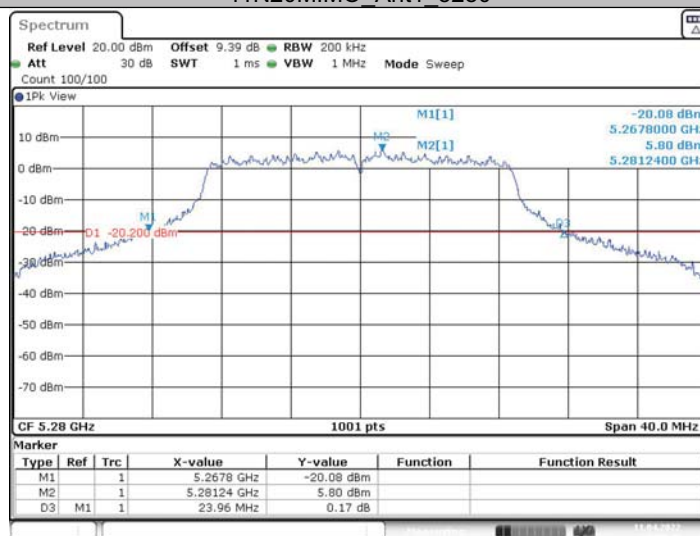
11N20MIMO_Ant1_5280
