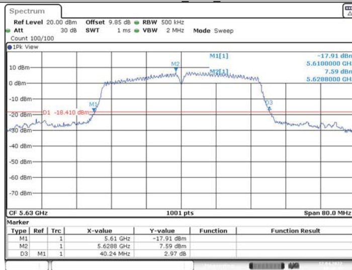
11N40MIMO_Ant2_5630
