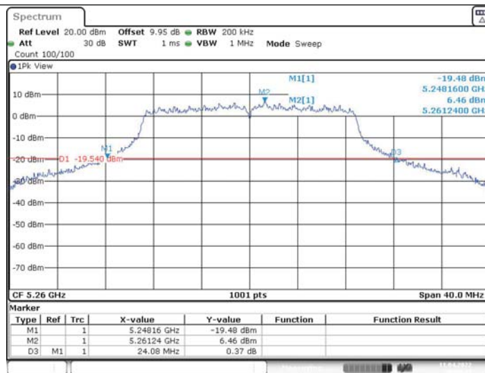
11N20MIMO_Ant2_5260
