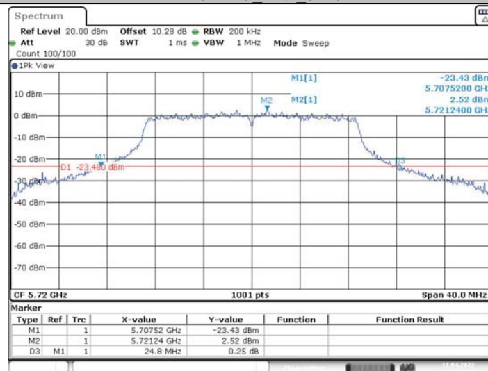
11N20MIMO_Ant1_5720
