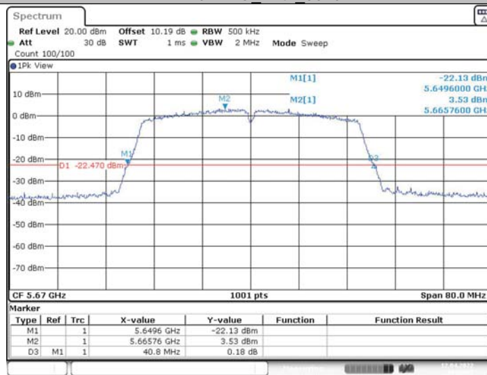
11N40MIMO_Ant1_5670
