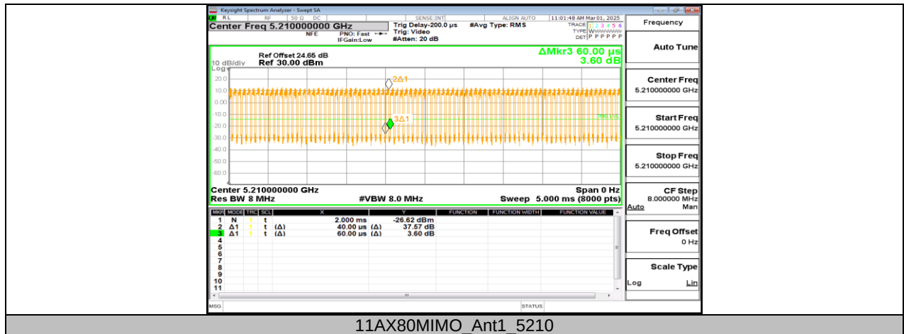
11AX80MIMO_Ant1_5210
