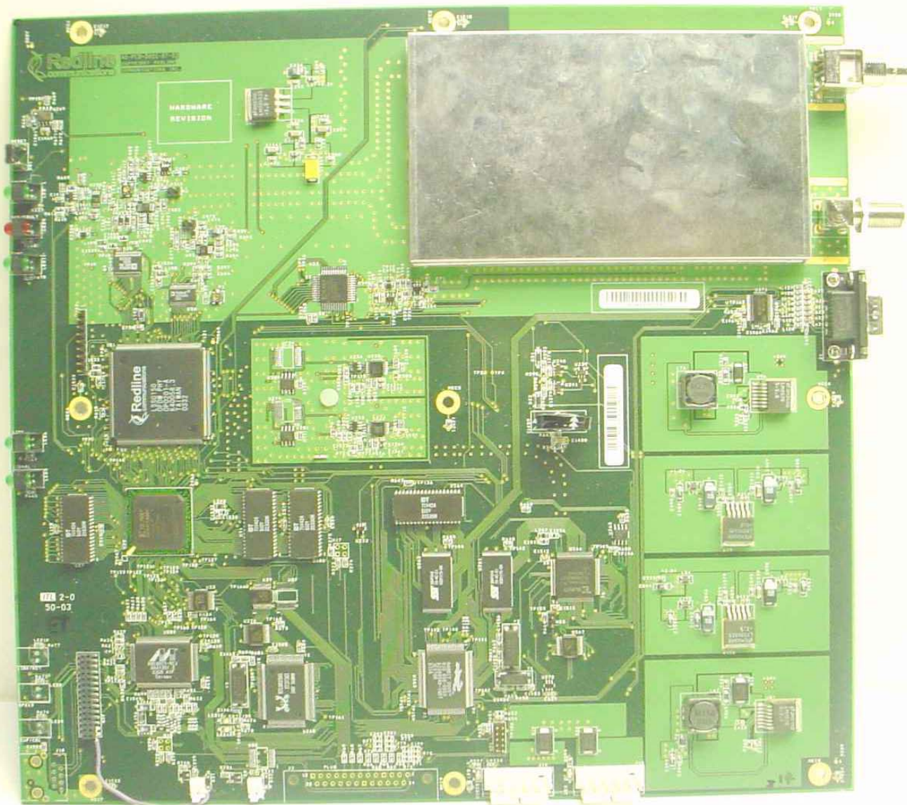
AN-50e / AN-30e Main Board
