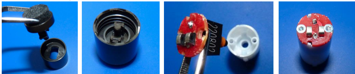
End Cap subassembly
