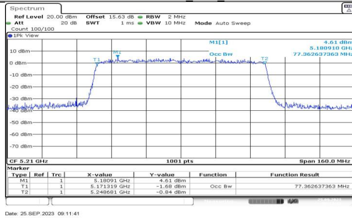
11AX80MIMO_Ant1_5210
