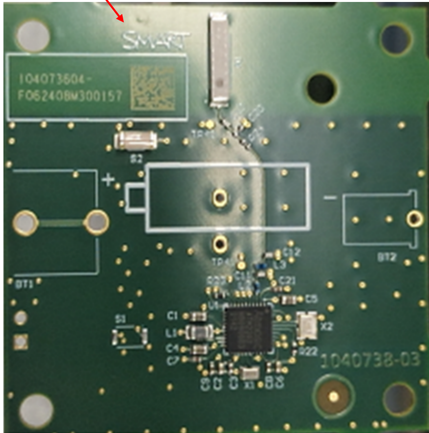
SRXMOD1 (Top)
