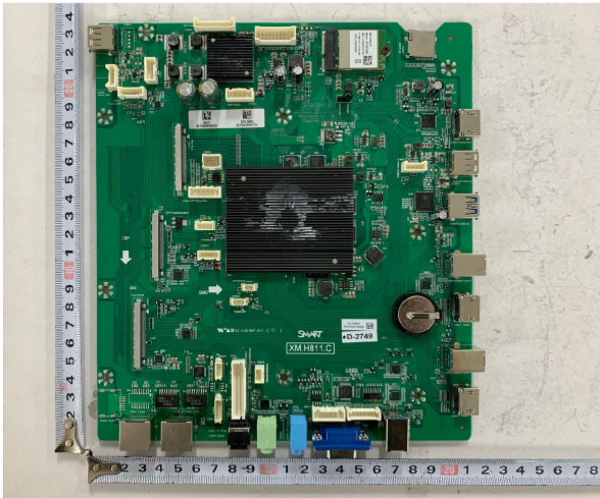
Casper Scaler PCB
