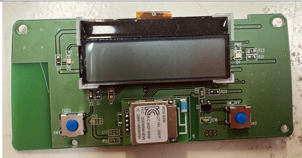
(SUB PCB_Front)
