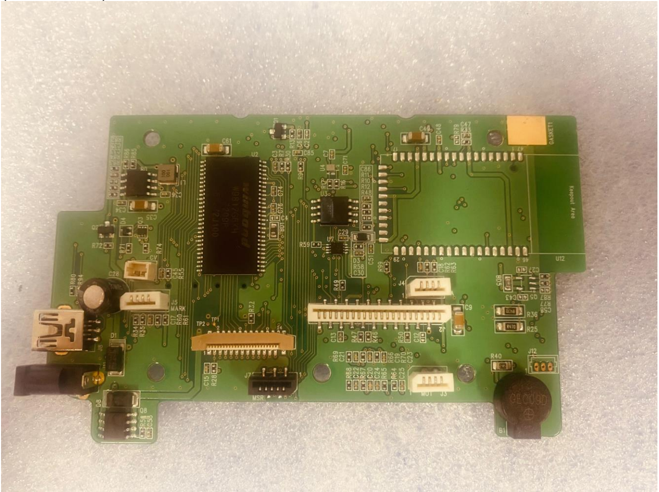
(MAIN PCB-1)
